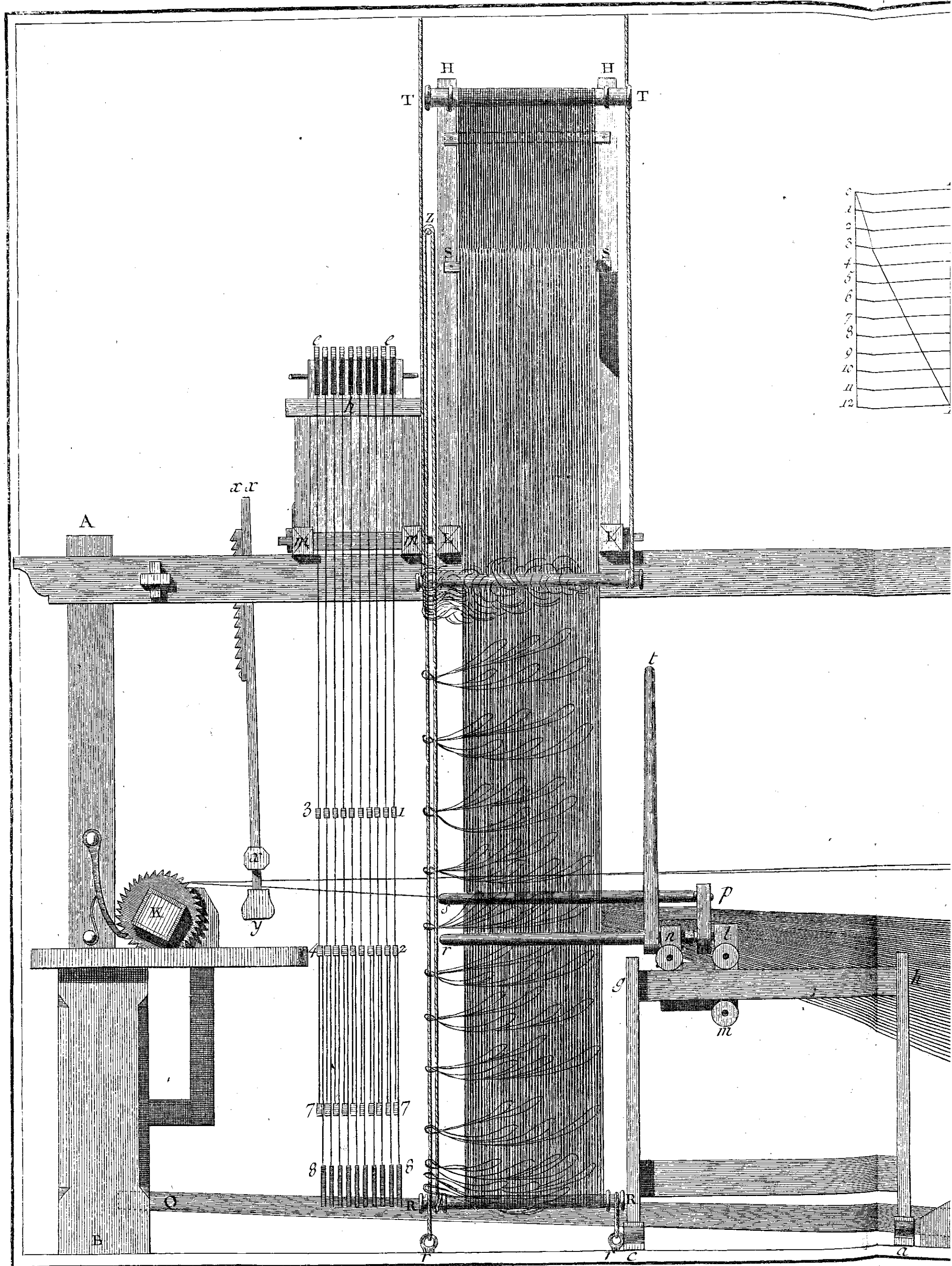
Soierie, Velours. Elevation Latérale du Métier pour fabrication.
