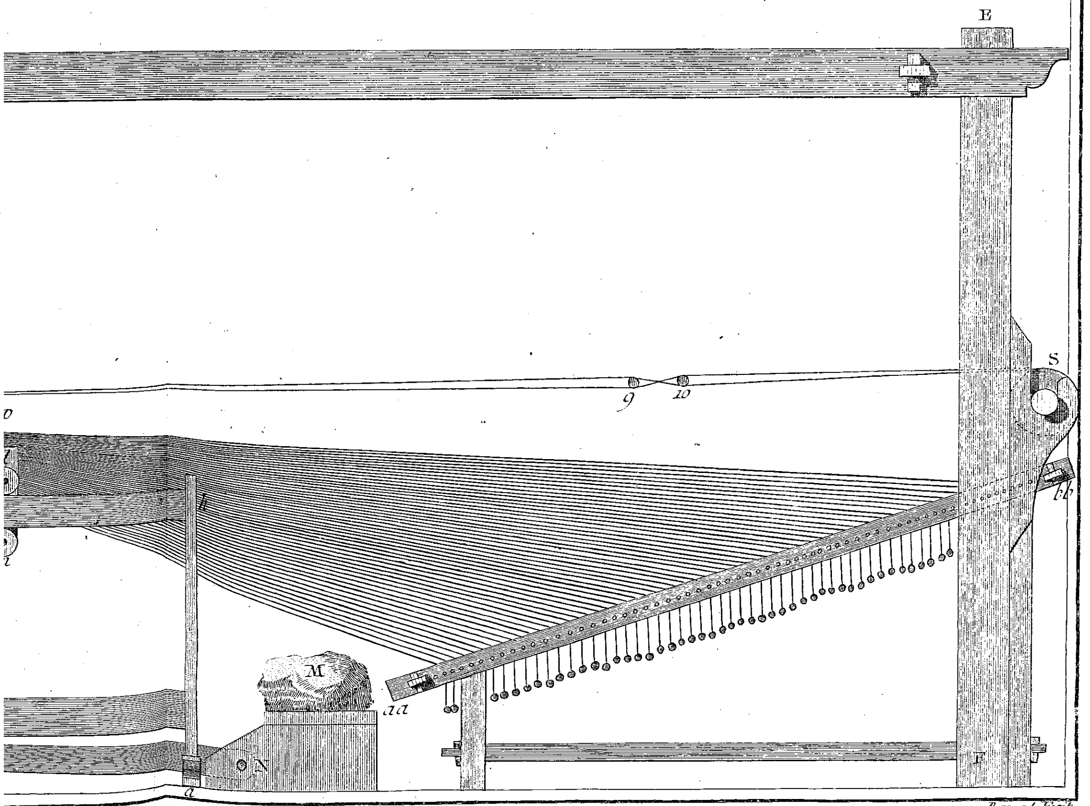
Métier pour fabriquer le Velours ciselé Vu dans l'instant qui precede celui de la Tire.
