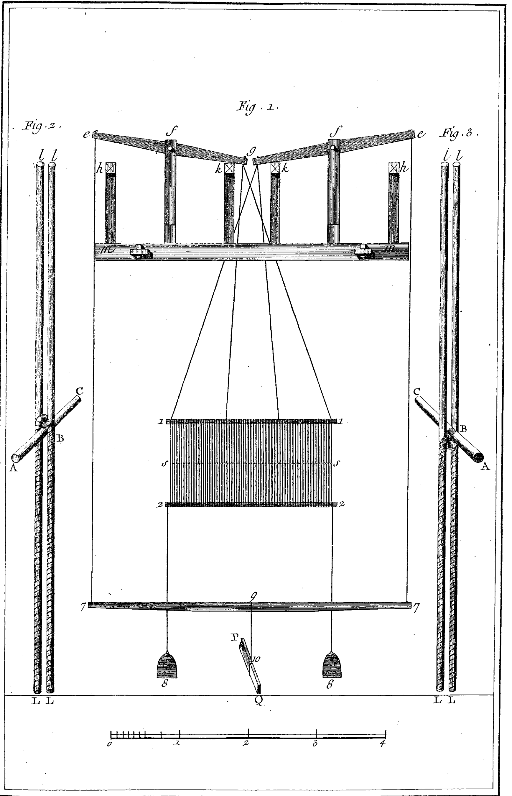
Soierie, Étoffes Brochées. Développement des Lisses de fond.
