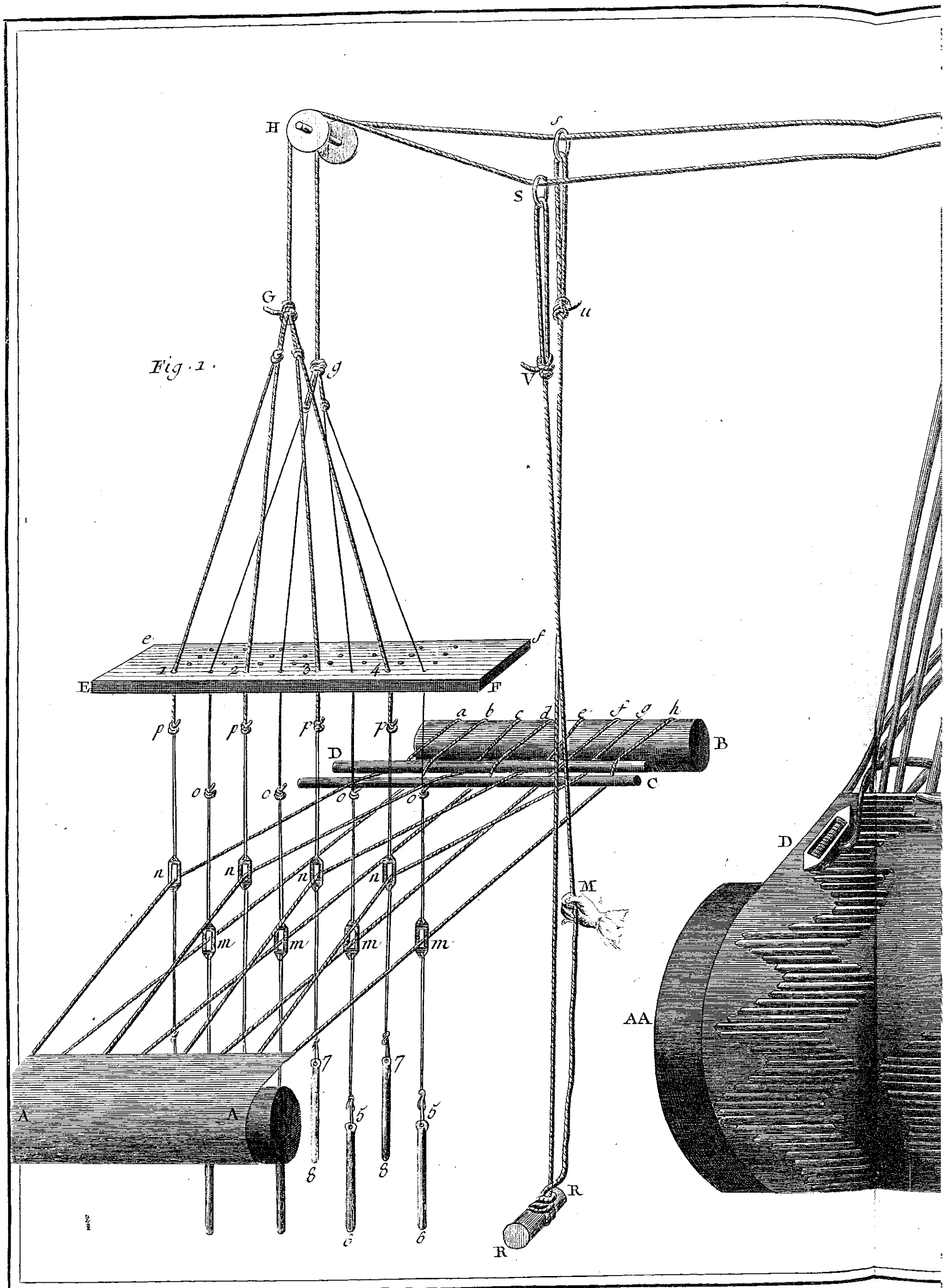
Soierie, Développement des Cordes de Rame et de Sangle Brochées ou le Poil des Velours frizés et Coupés, Partie l'Étoffe.
