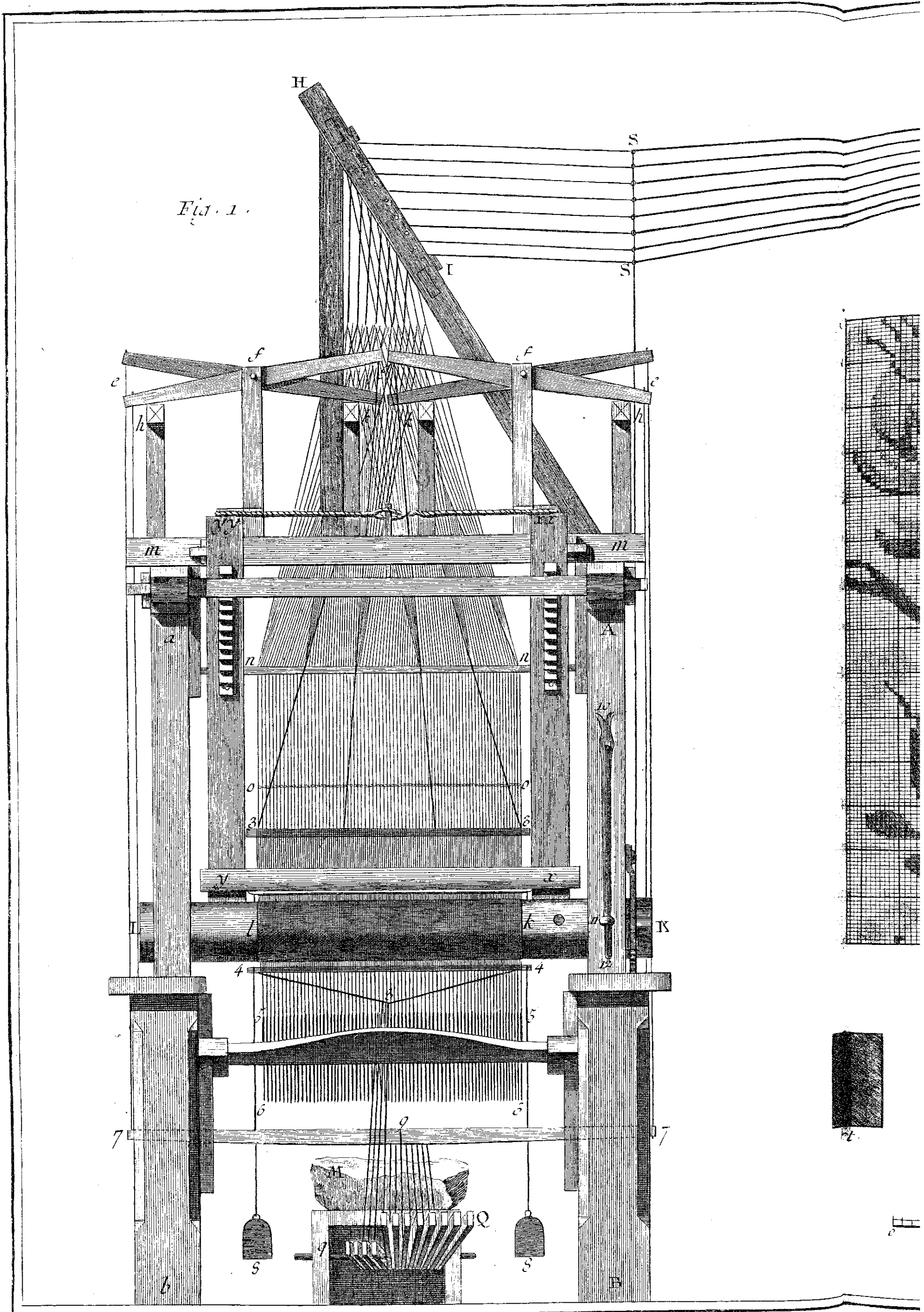
Soierie, Étoffes Brochées, Élévation Géométrale du deva
