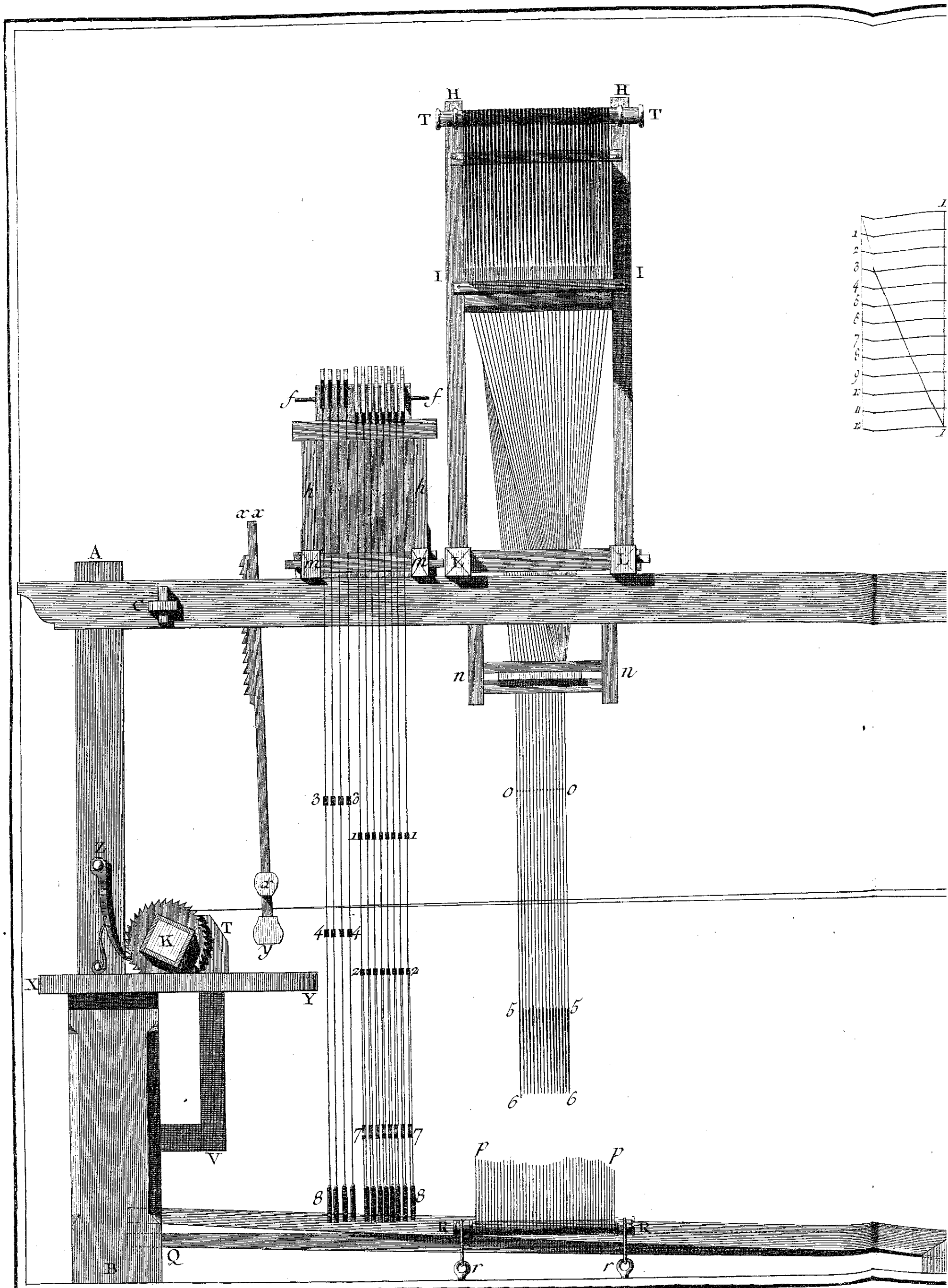
Soierie, Étoffes Brochées Élévation Latérale du Mé.
