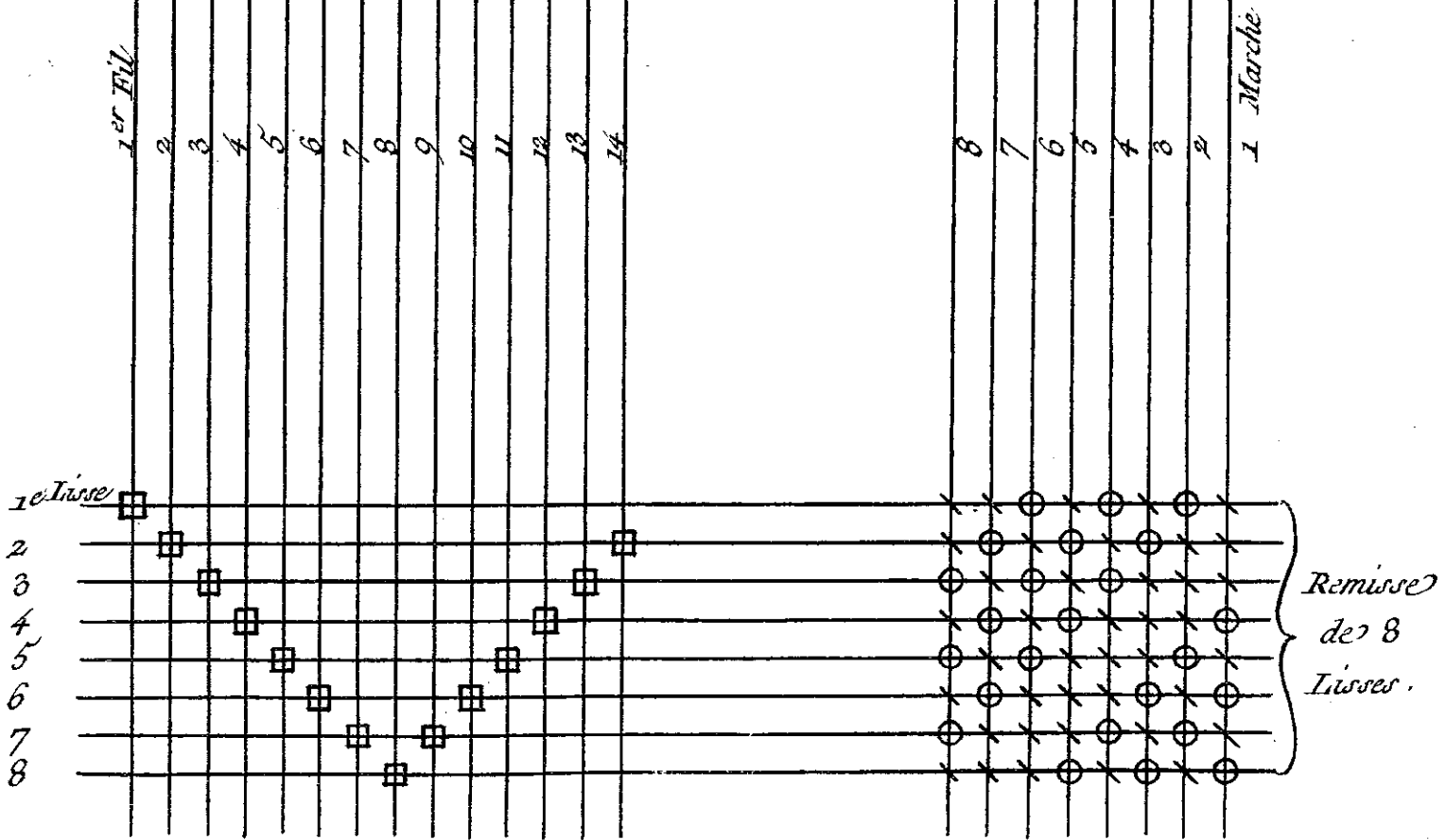
Course de 14 Fils sur 8 Lisses par le moyen du Retour.
