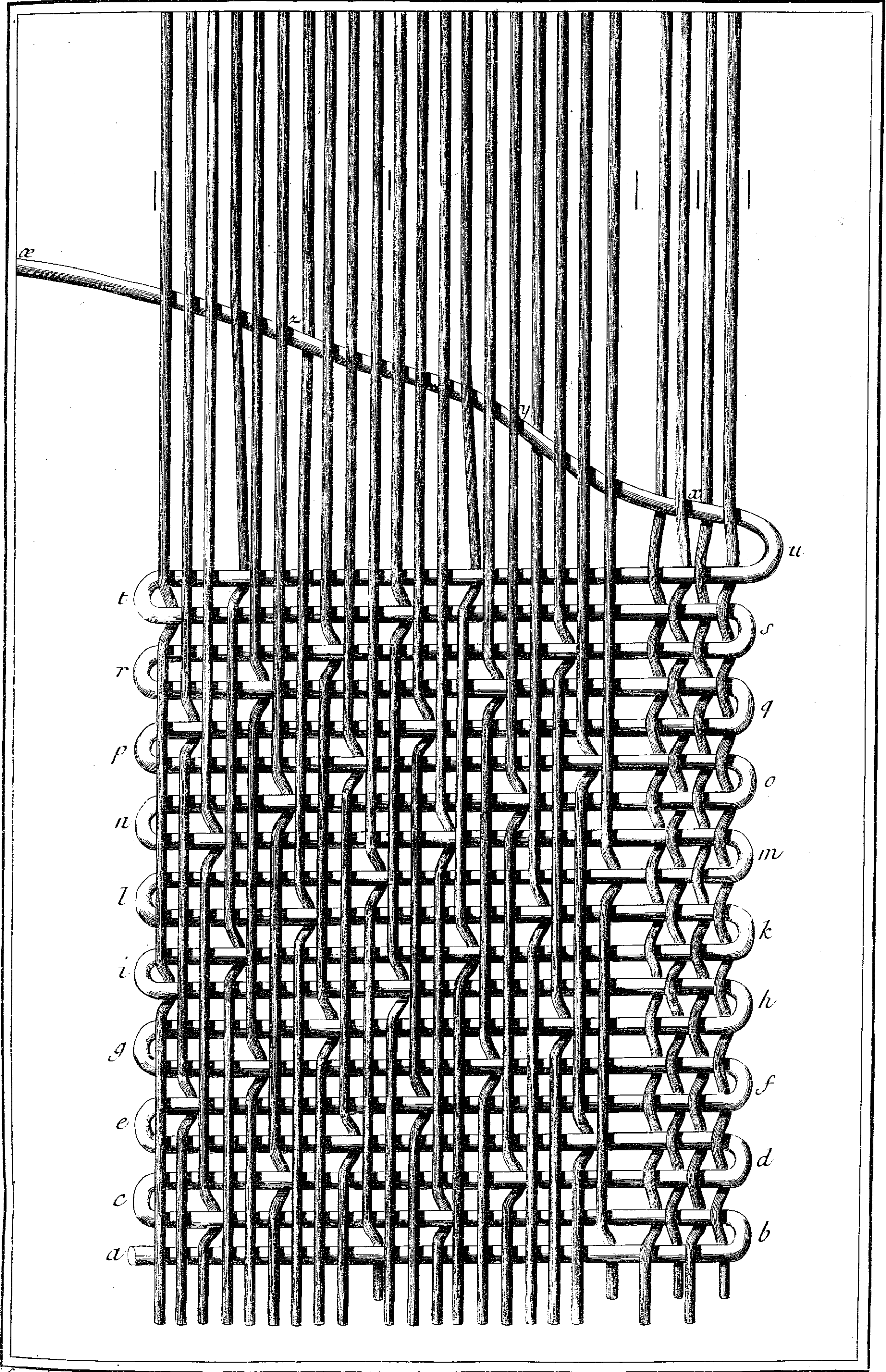
Soierie, Etoffes en Plein, Satin à dix Lisses Vu du coté de l'endroit. f
