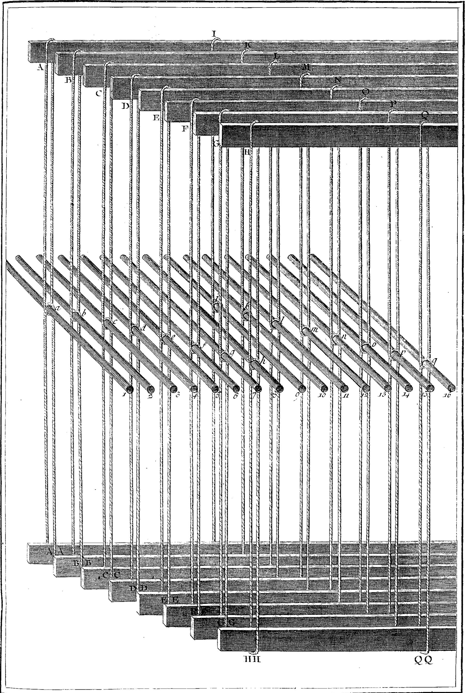
Soterie, Remetage ou Passage des Fils de la chaîne dans les Lisses.
