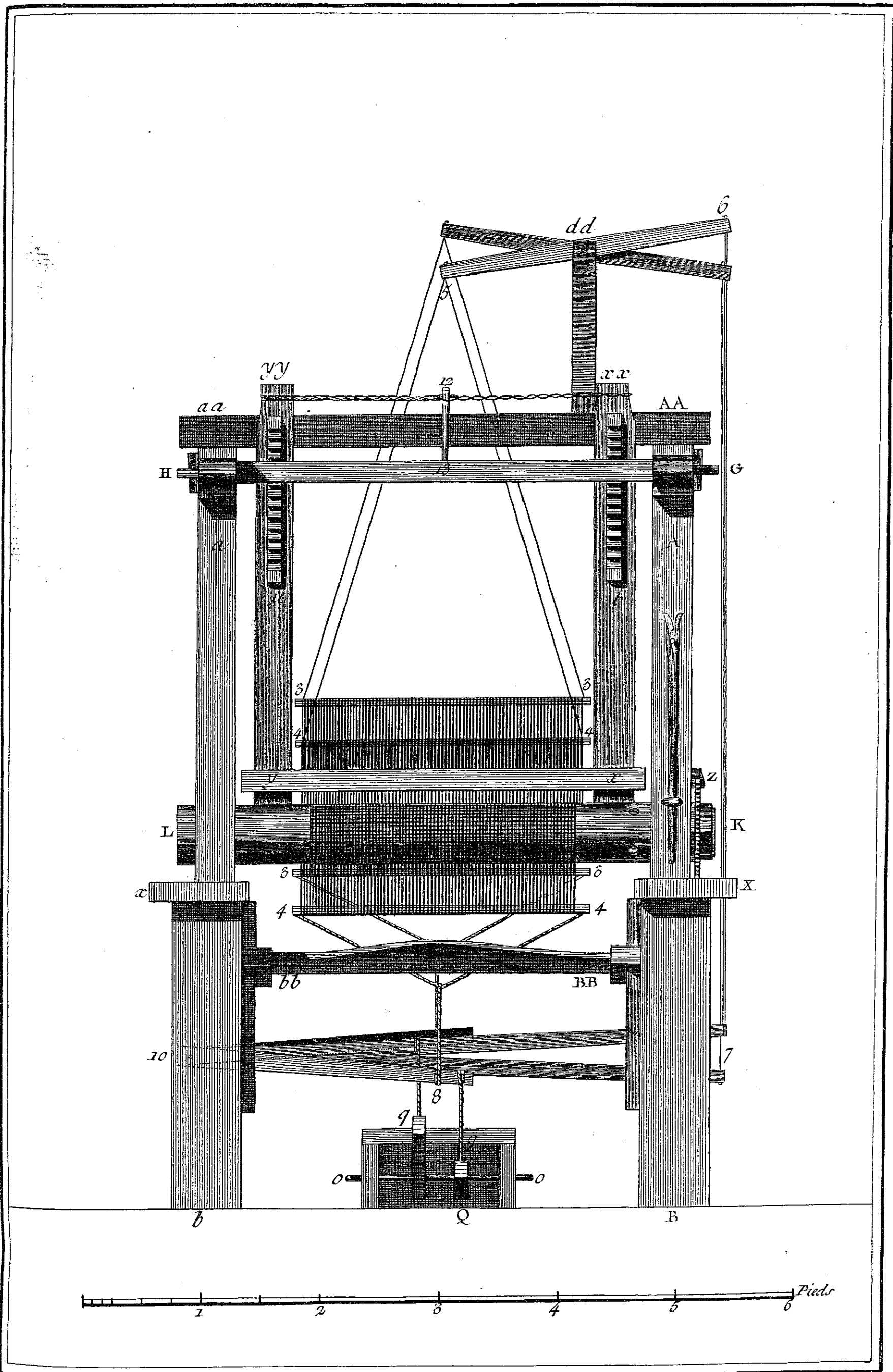
Soierie, Élévation Géométrale de la partie antérieure. du Métier pour fabriquer les Étoffes unies, comme Taffetas, Satin, et Serge.
