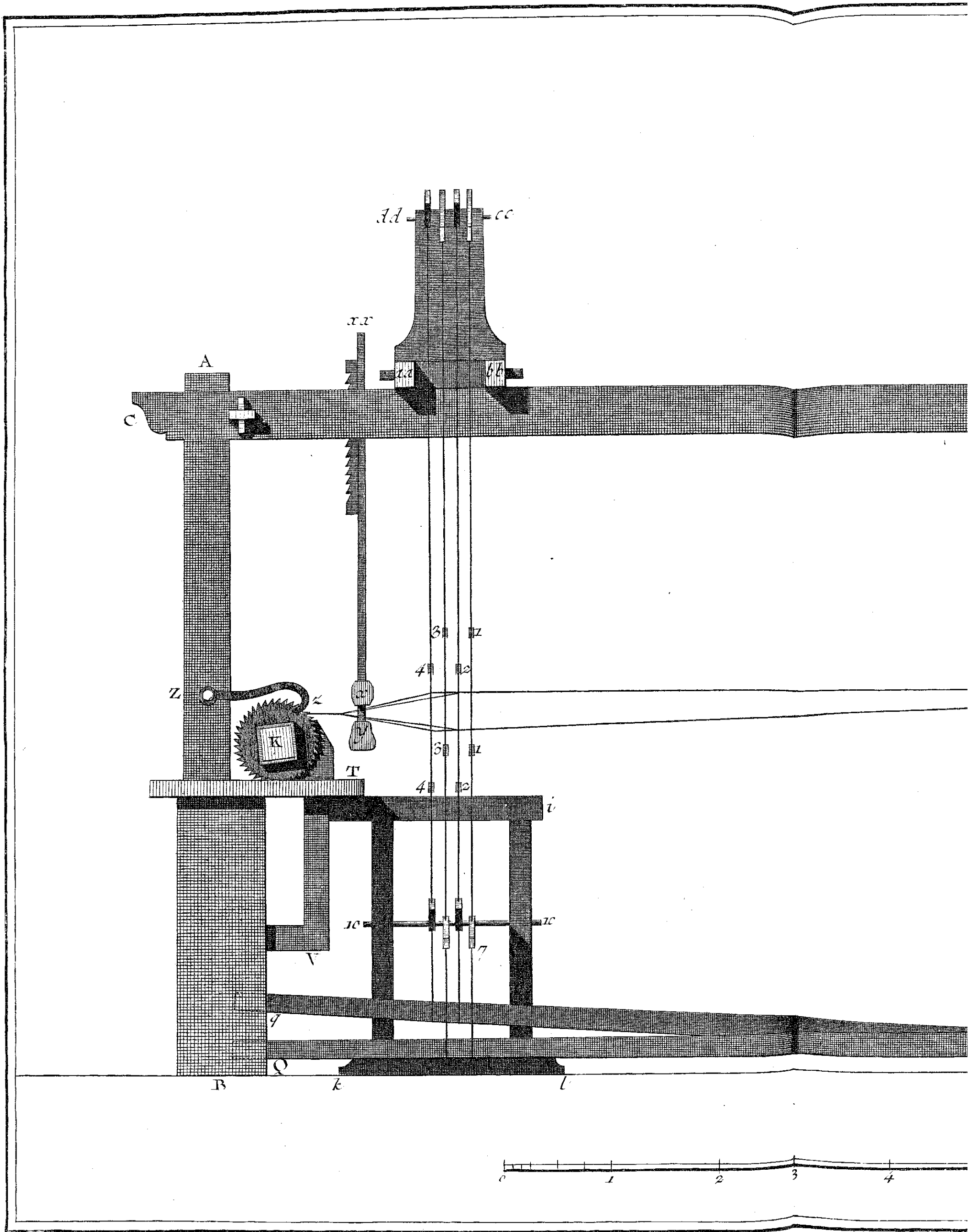
Soierie, Elevation Géométrale de la partie Latérale du Métier pour fab
