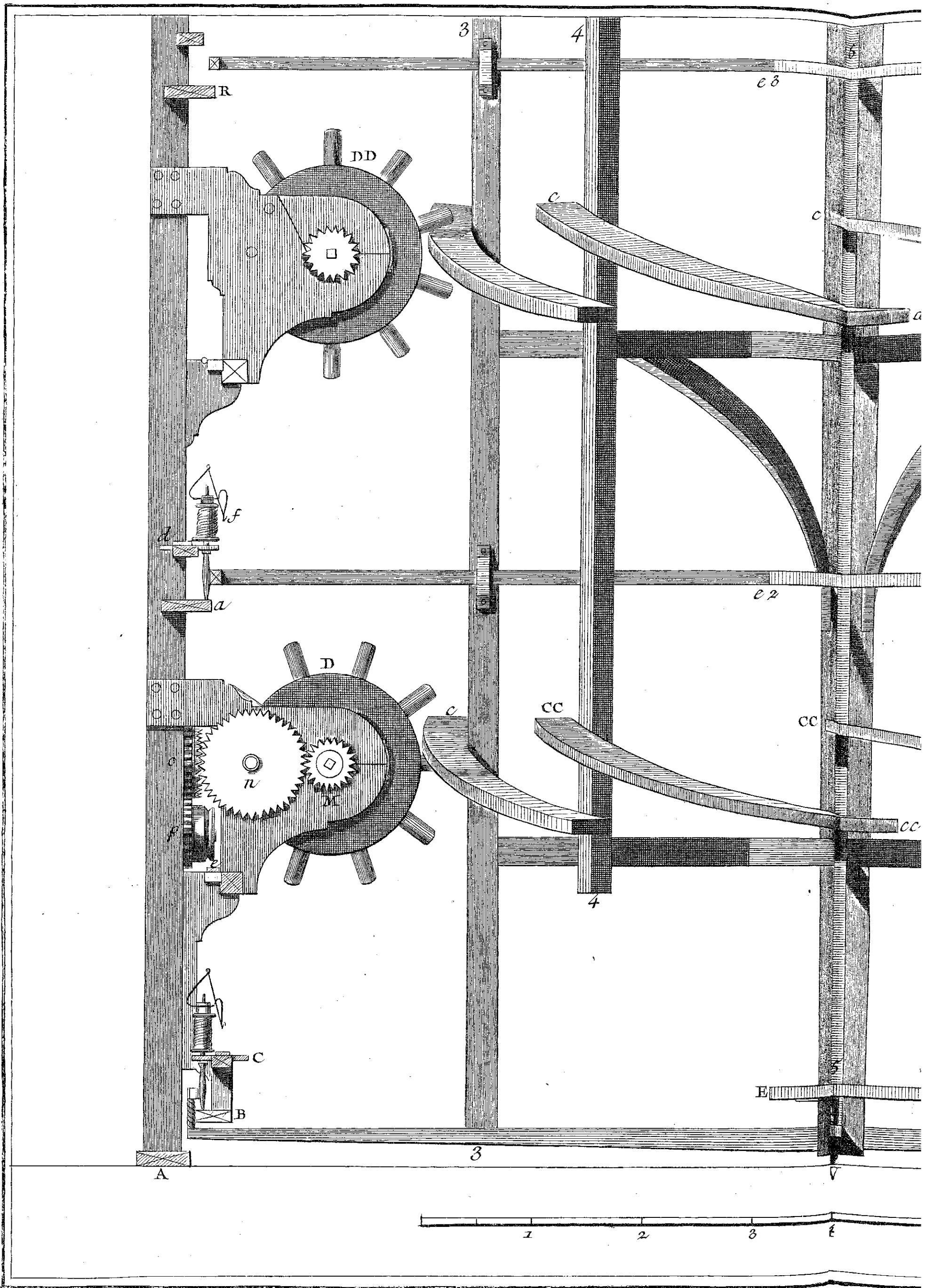
Soierie, coupe Diamétrale du Moulin de Piémot et Élev.
