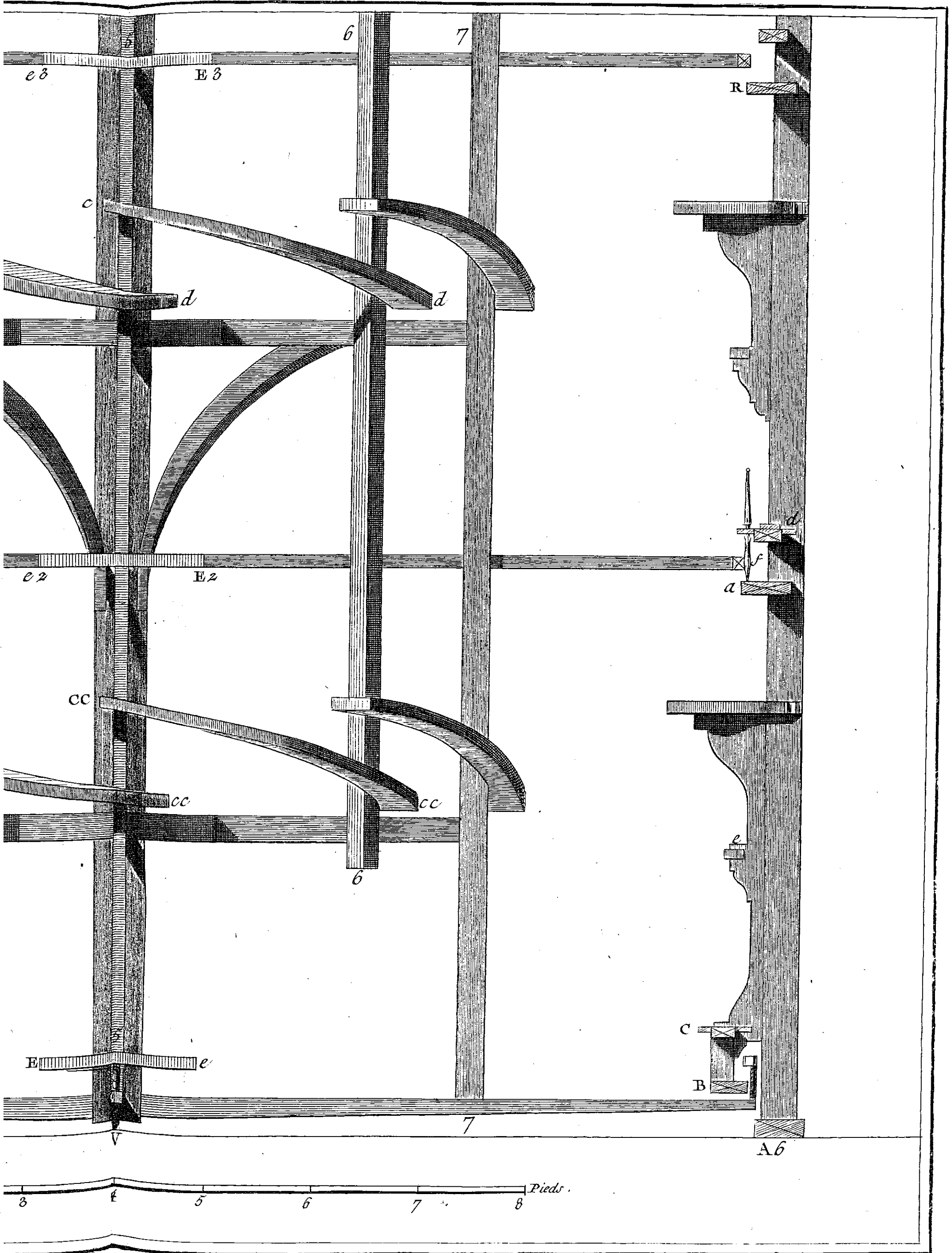
De Piémont et Élévation de la Lanterne qui est dans l'Intérieur.
