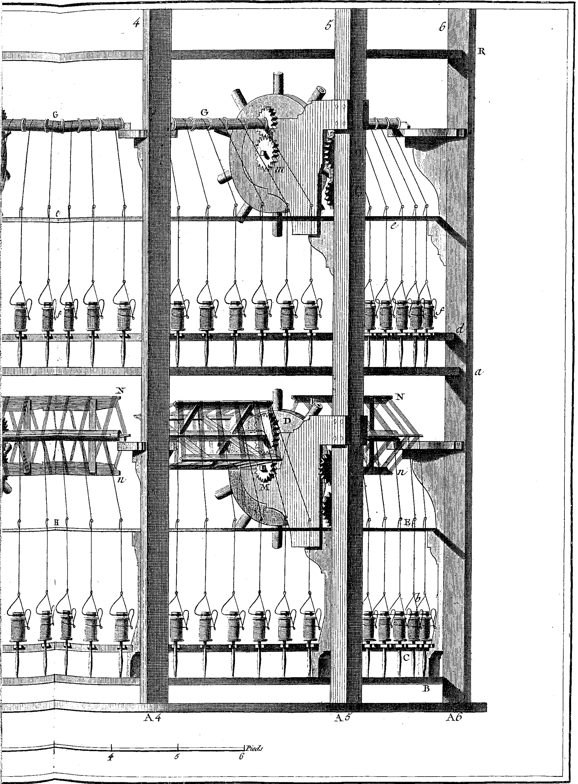
ralle du Moulin de Piemont, pour Organiser les Soies.
