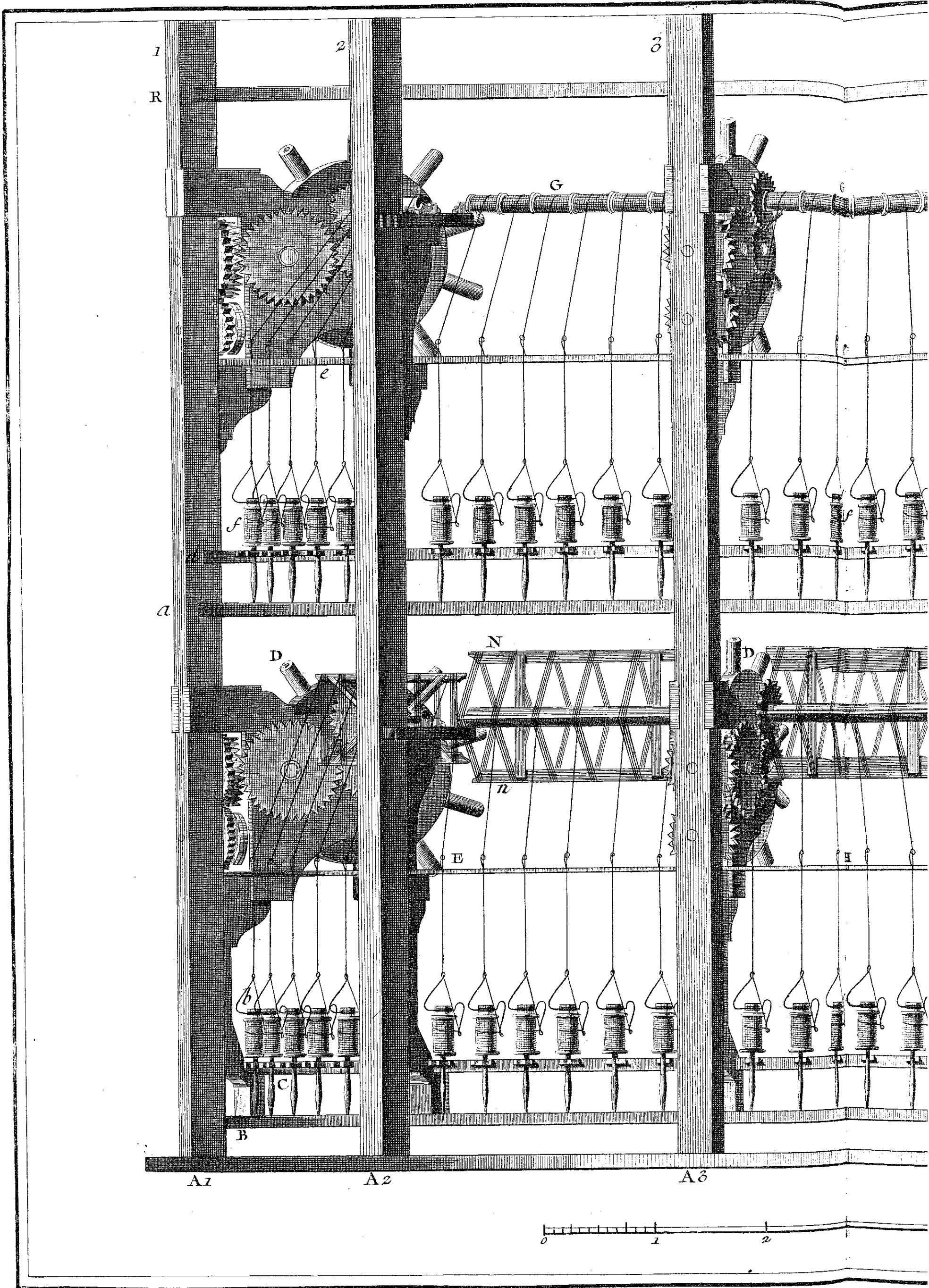
Soierie, Elevation Géométrale du Moulin
