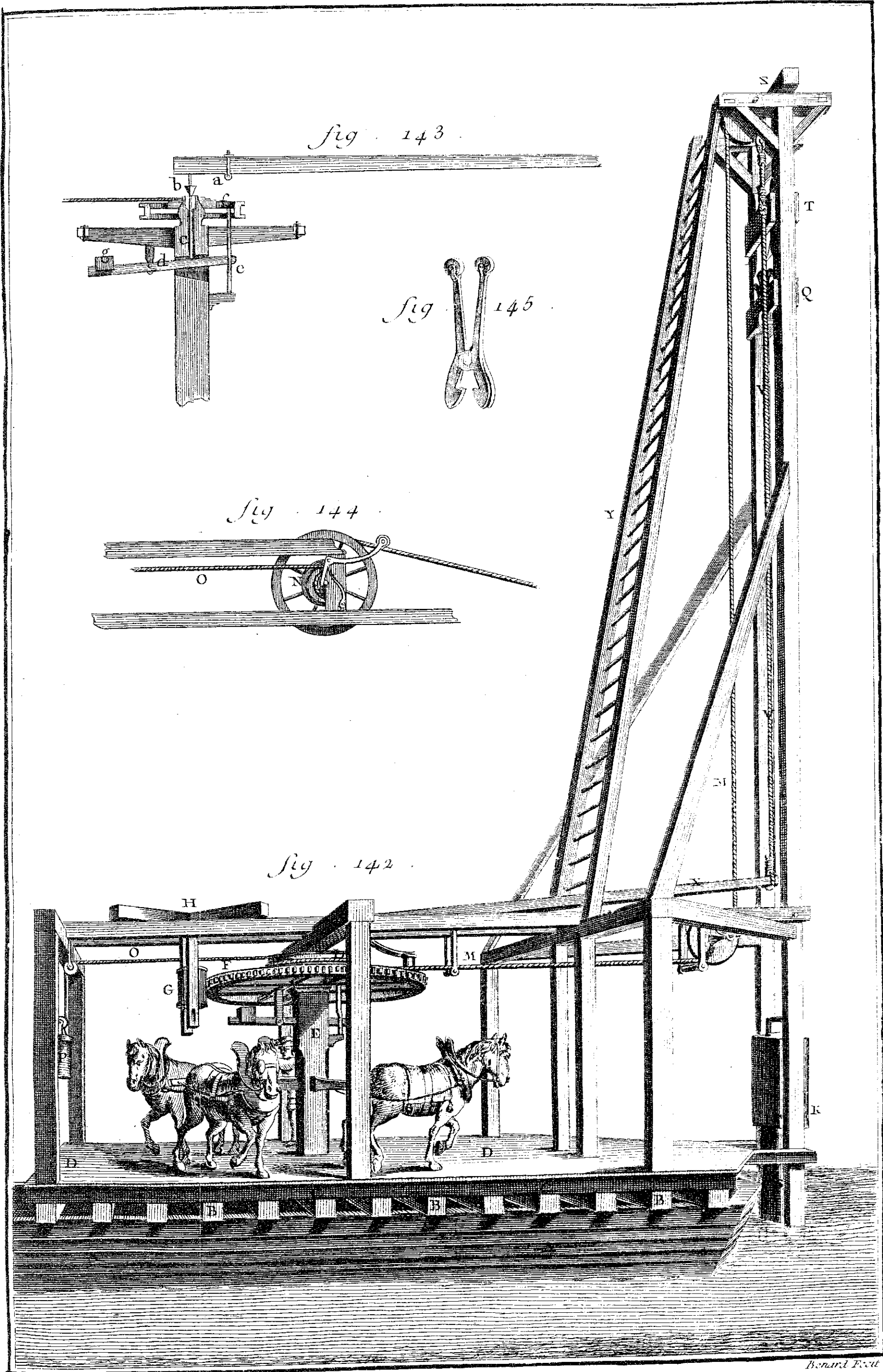
Charpente Mouton a cheval sur bateaux
