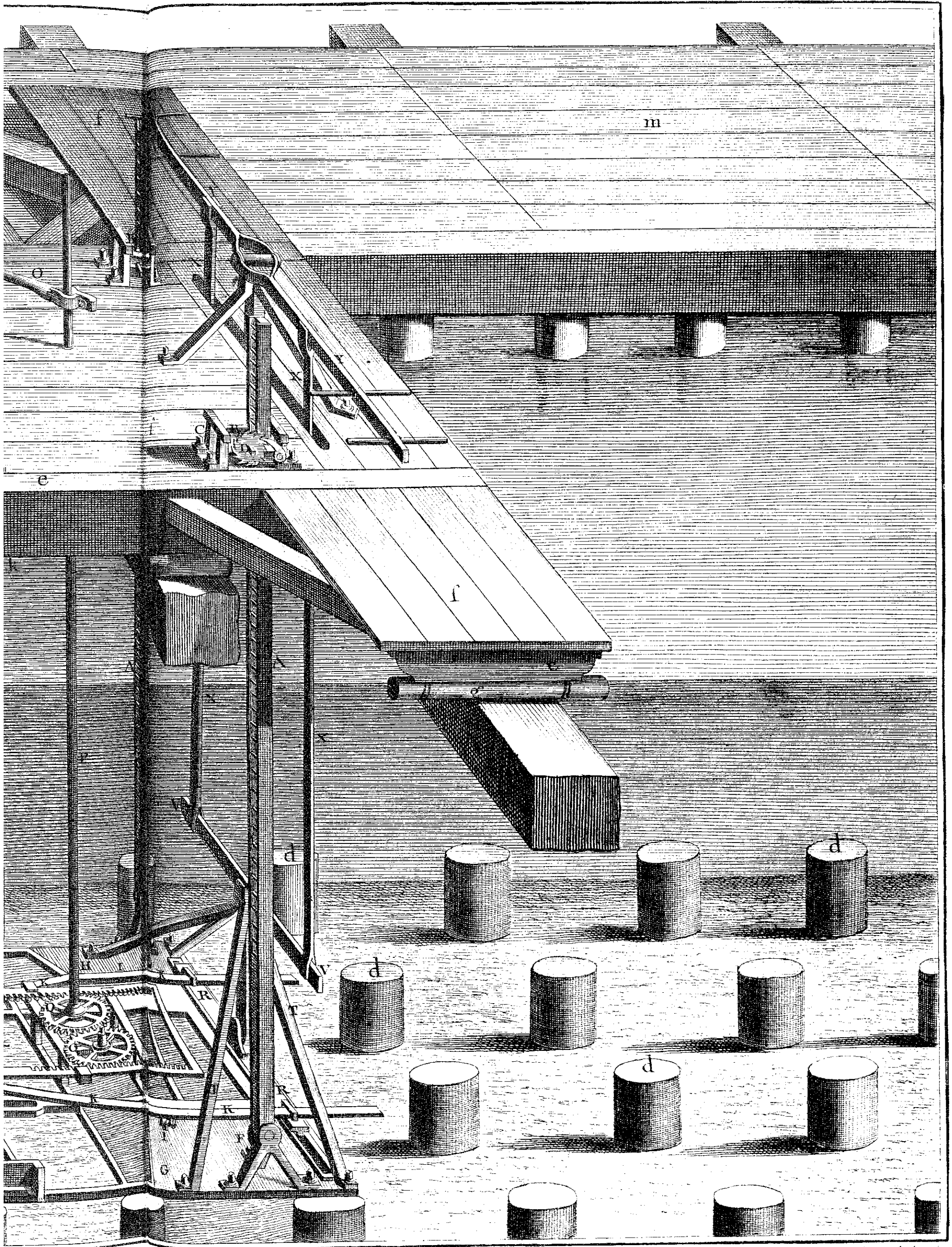
Charpente, Machine à scier dans l'Eau.
