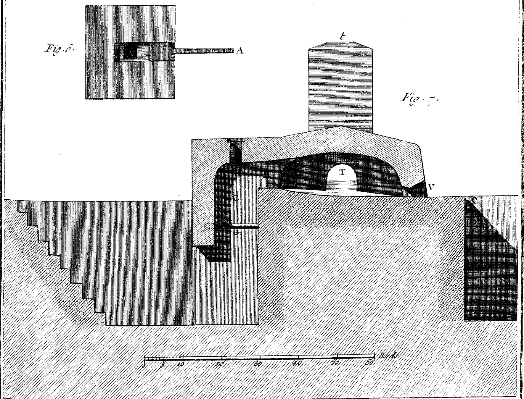
Fontes des Cloches, Coupes Transversale et Longitudinale du Fourneau.
