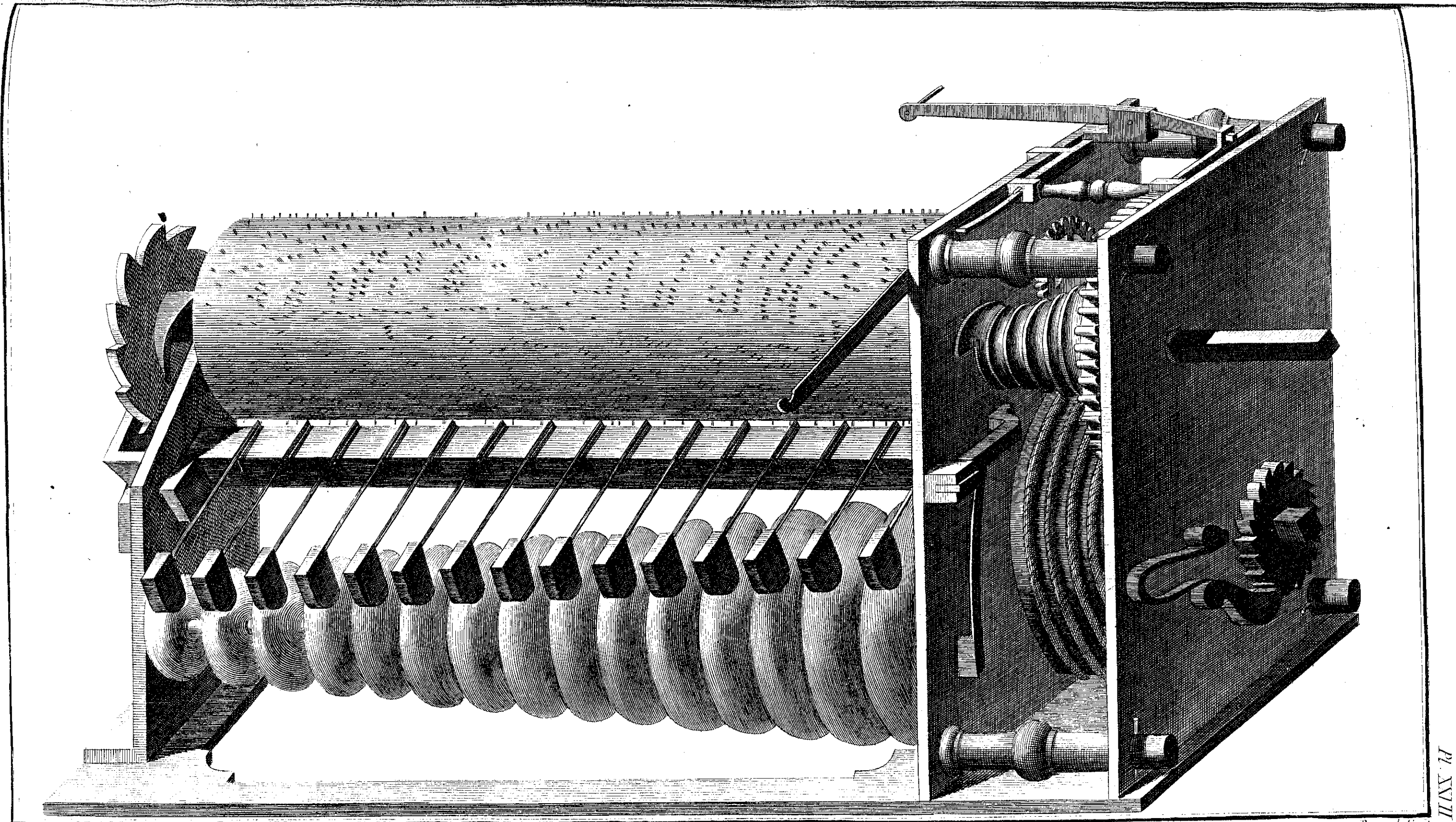
Horlogerie, Vue perspective d'un Carillon.
