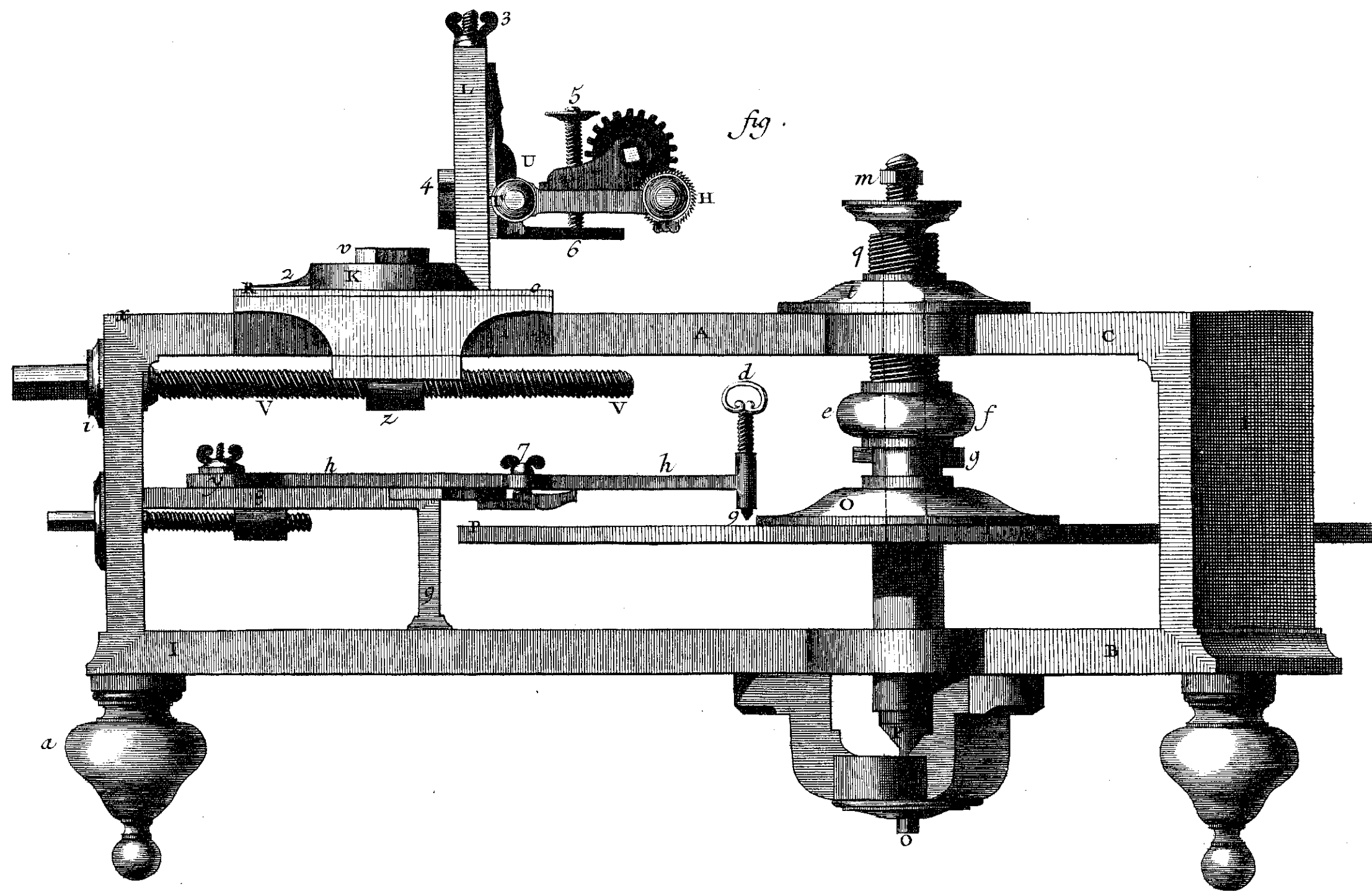
Horlogerie, Profil de la Machine du Sieur Hulot pour fendre les Roues.
