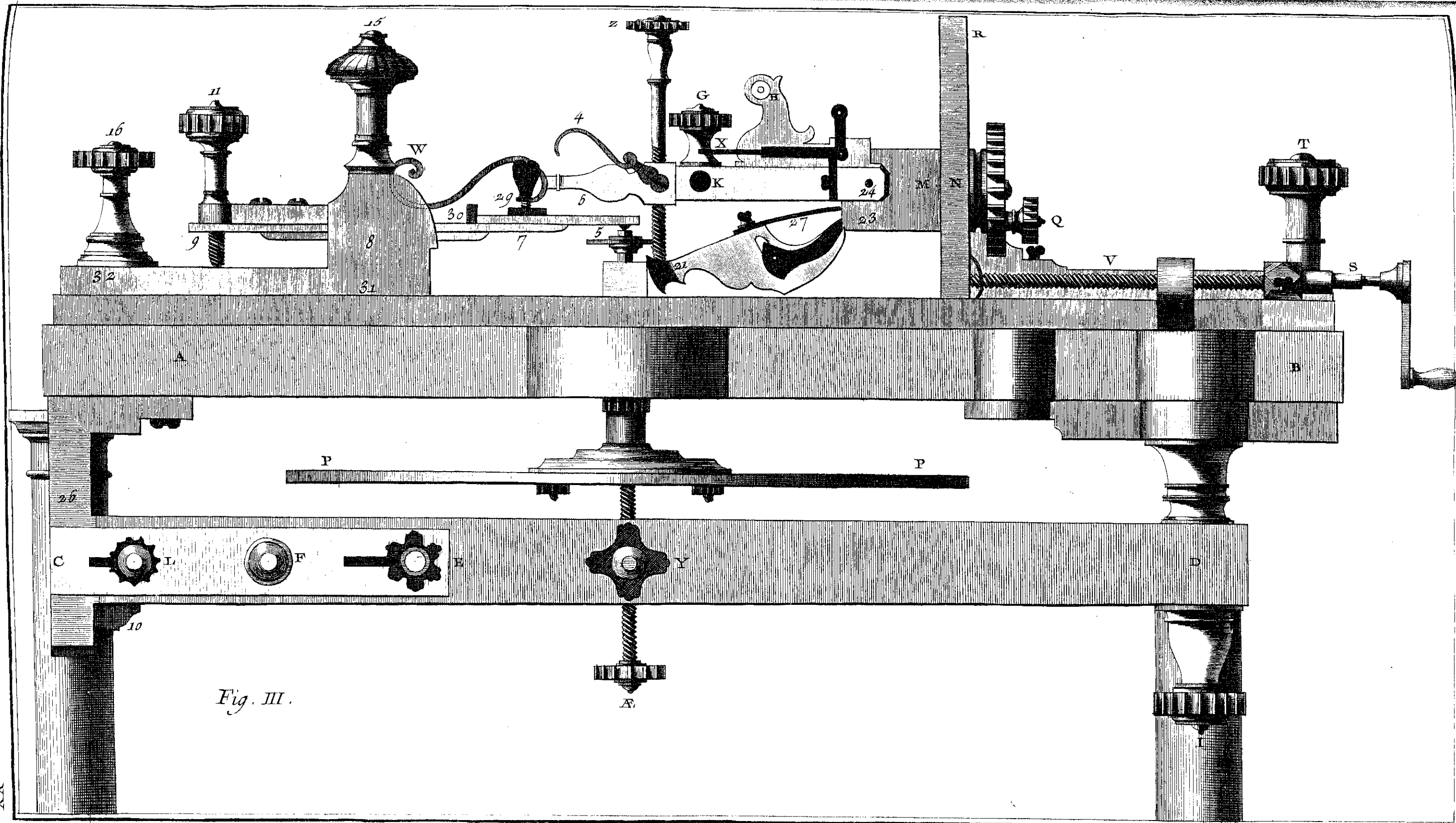
Horlogerie, Profil de la Machine de Sulli pour fendre les Roues.
