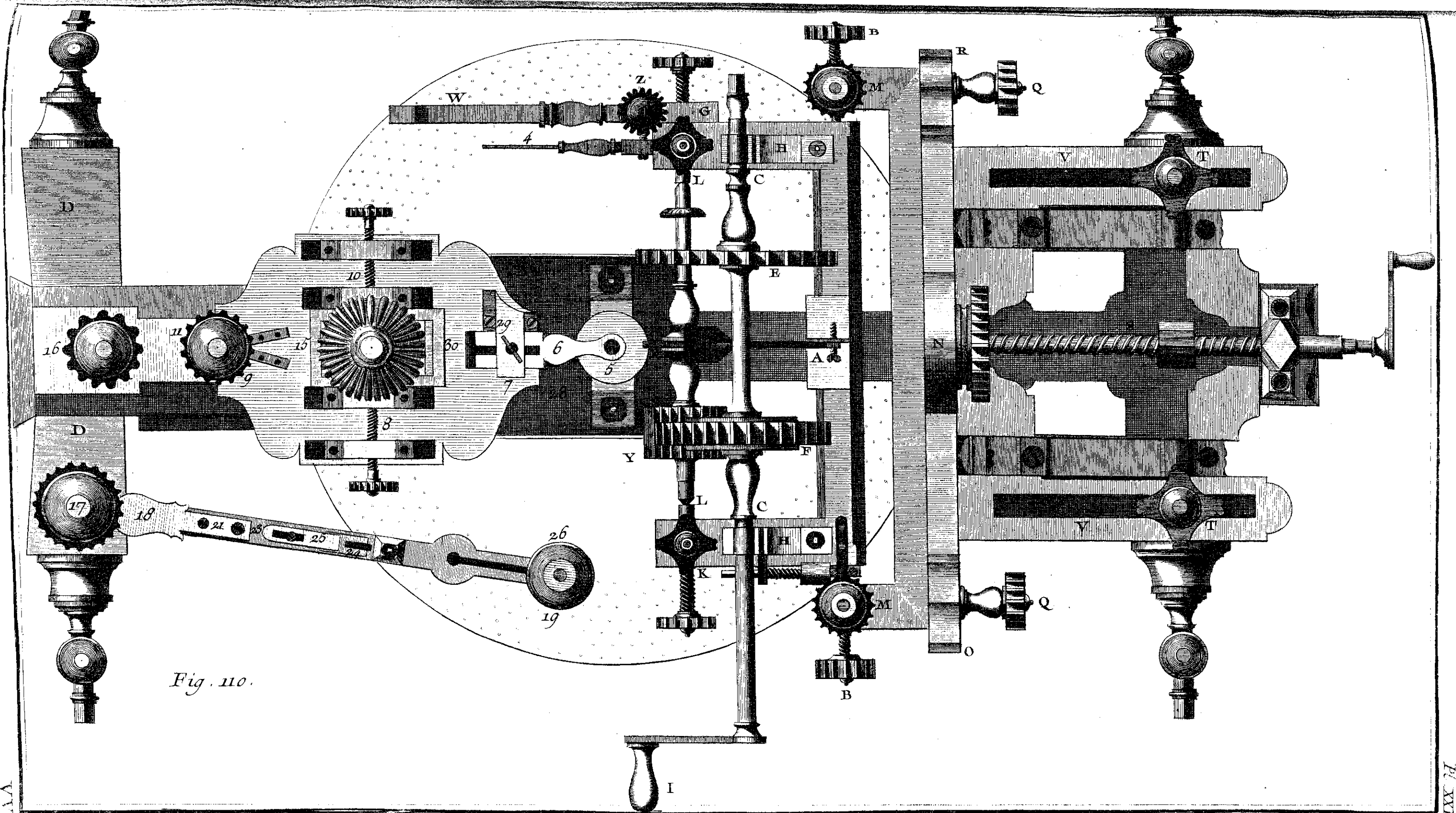
Horlogerie, Plan de la Machine de Sulli pour fendre les Roues.
