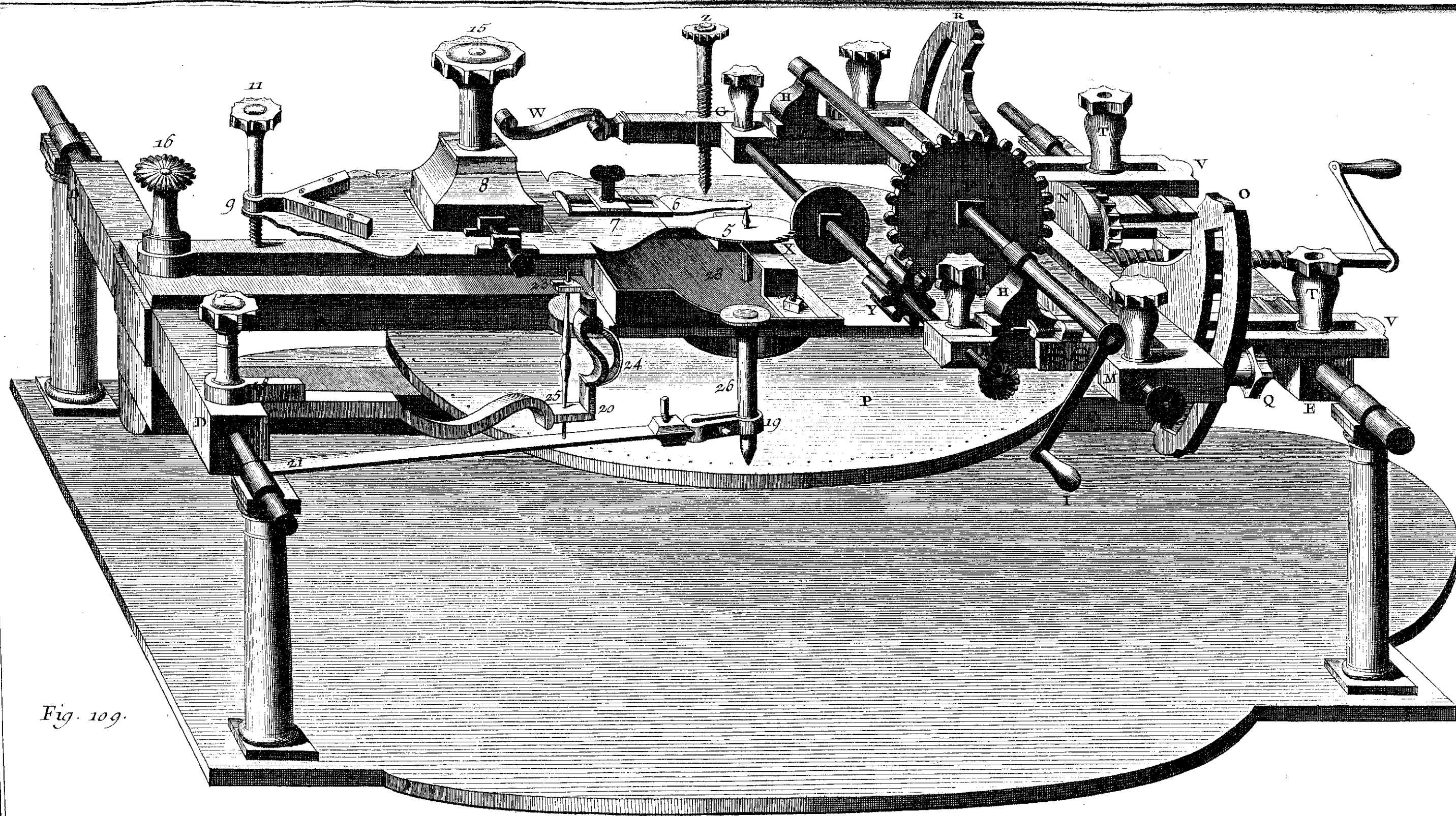
Horlogerie, Vue perspective de la Machine de Sulli pour fendre les Roues.
