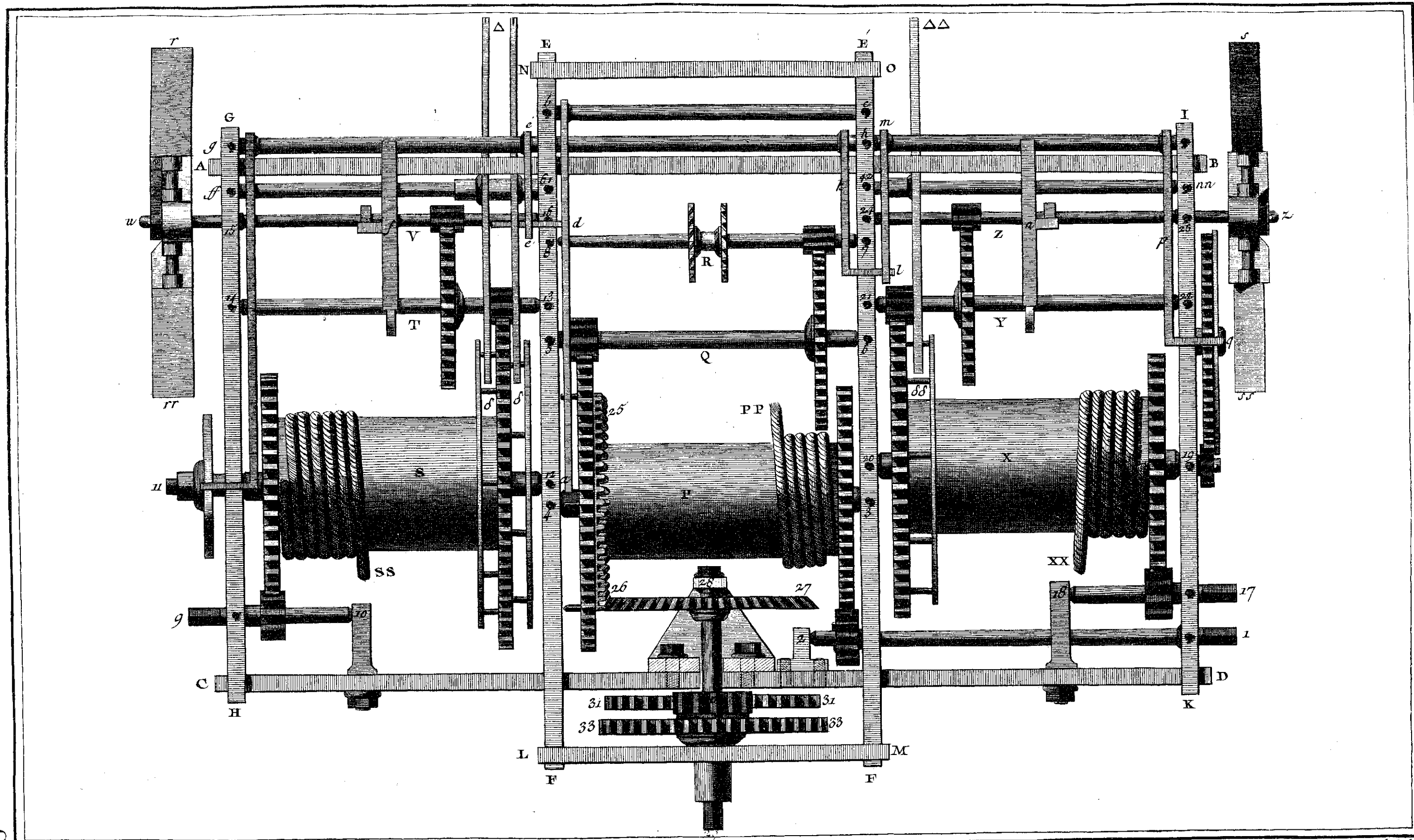
Horlogerie, Plan de l'Horloge Horizontale.
