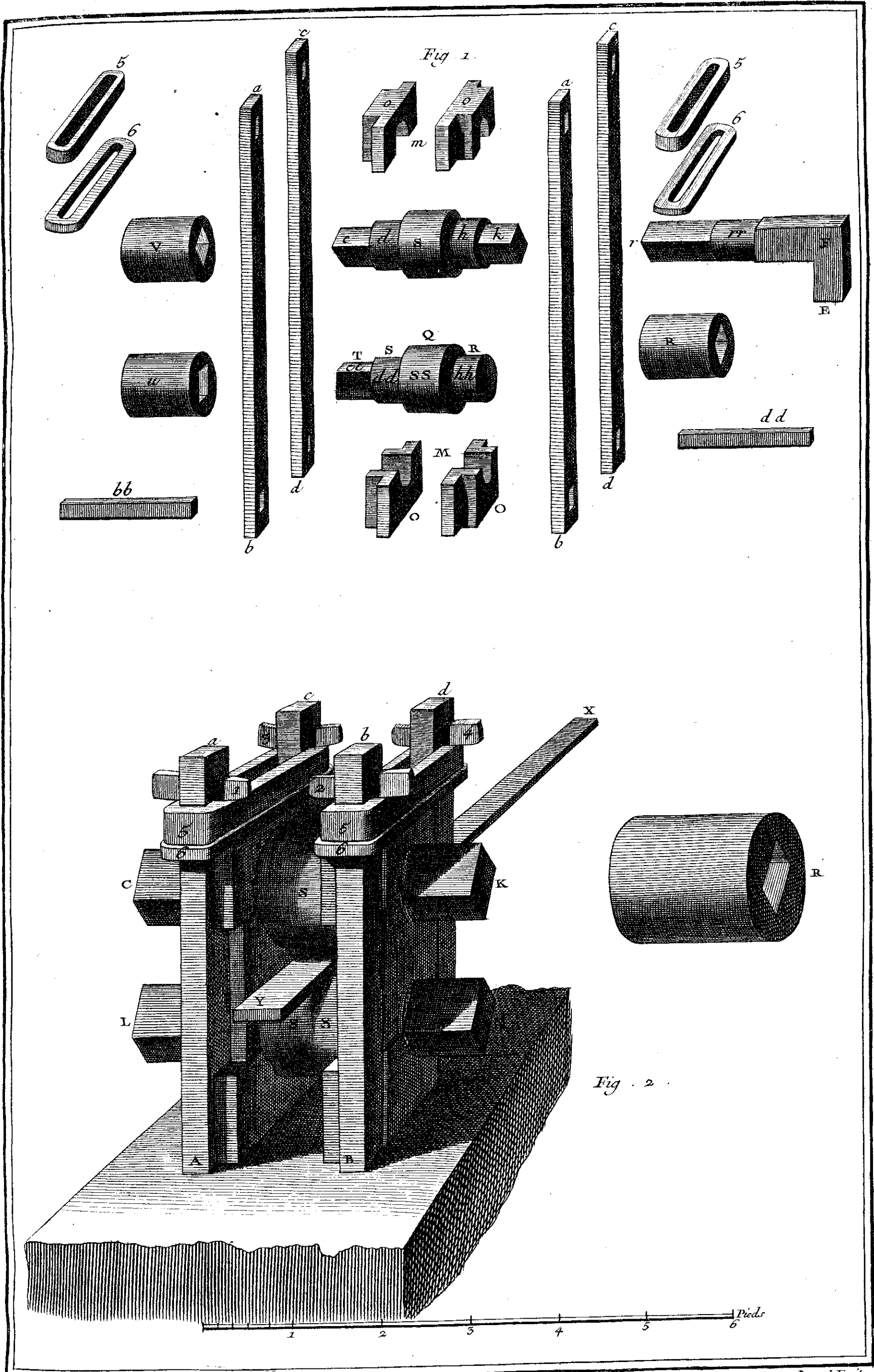
Forges. 5. Section, Fenderie, Developpemens des Espatars.
