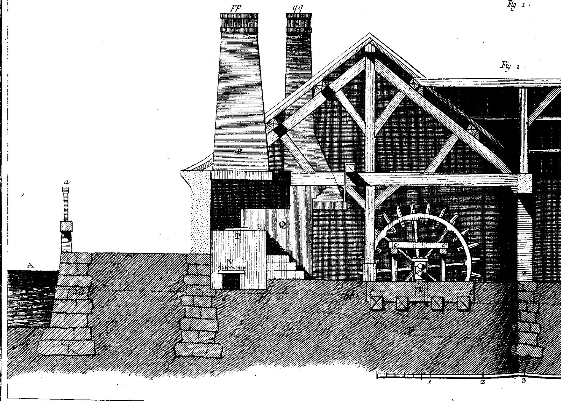
Forges. 5 e Section, Coupes Transversalle et Longitudinale
