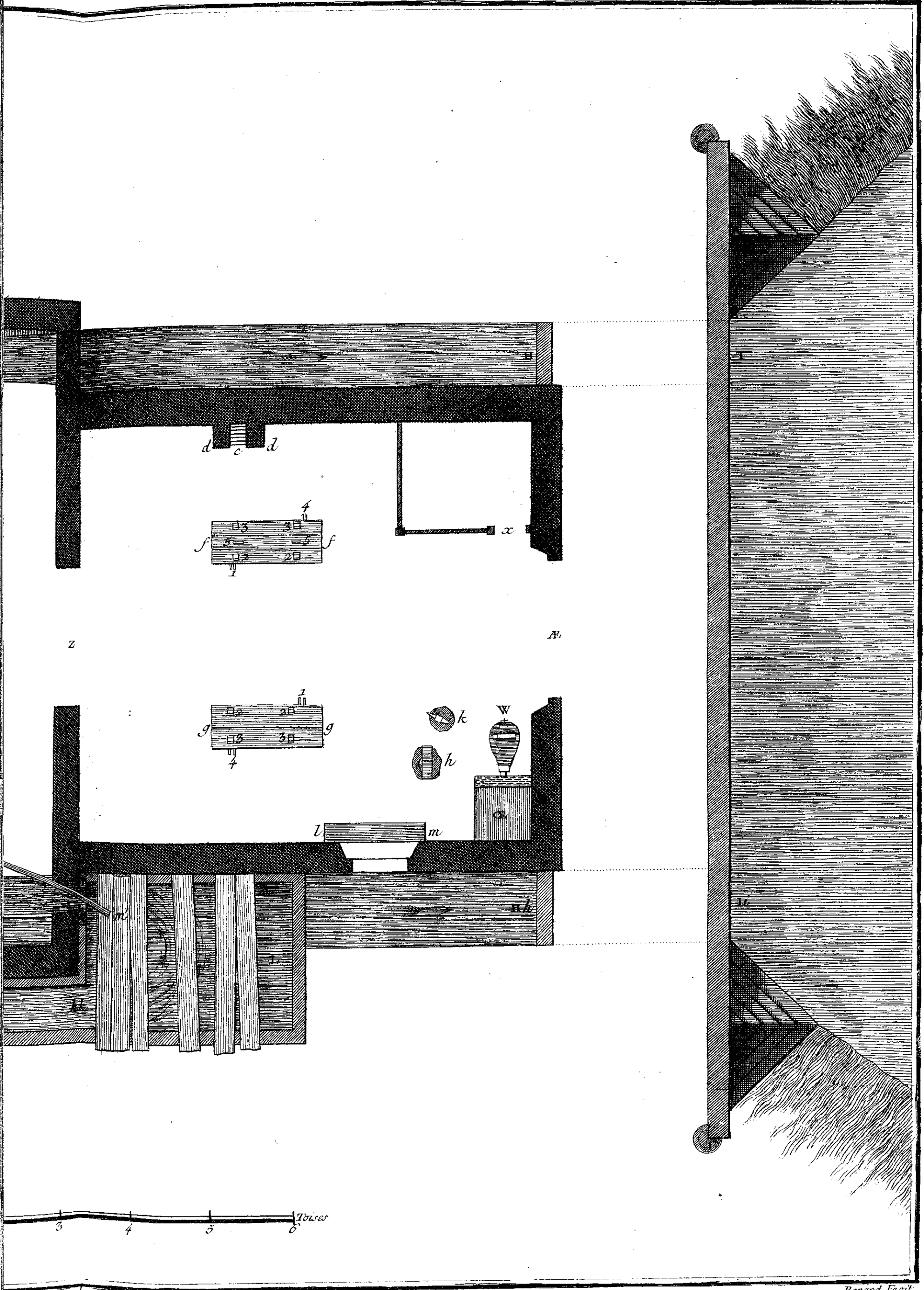
en Général d'une Fenderie.
