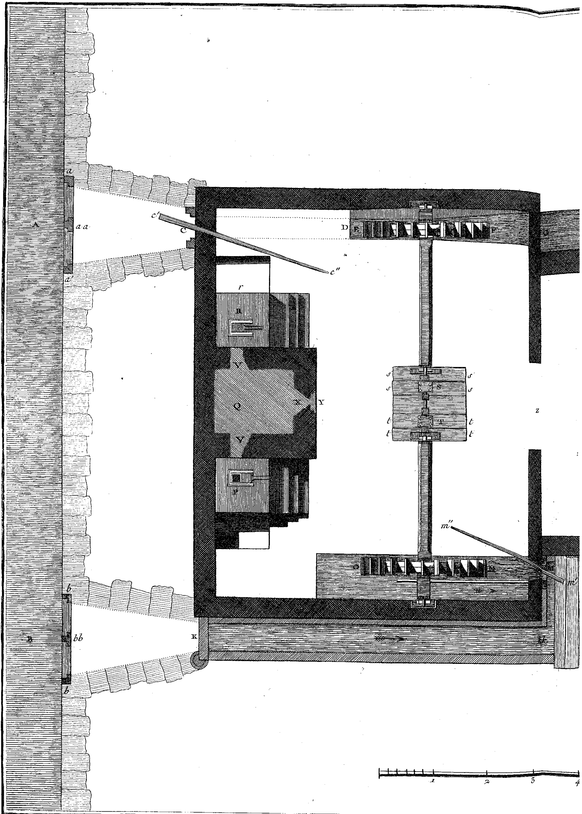
Forges, 5 e Section. Plan Général d'une.
