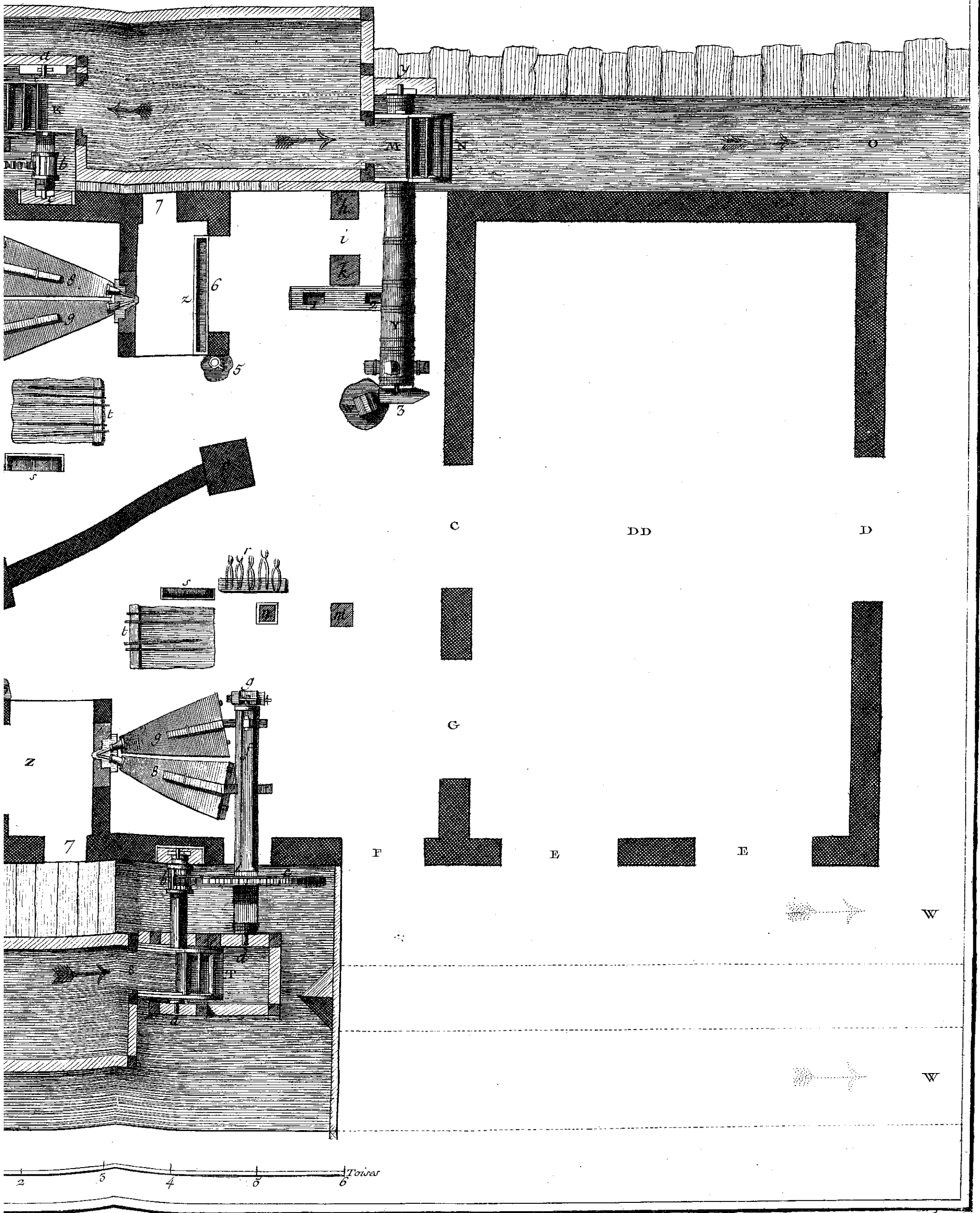
Plan Général d'une Forge à deux Feux.
