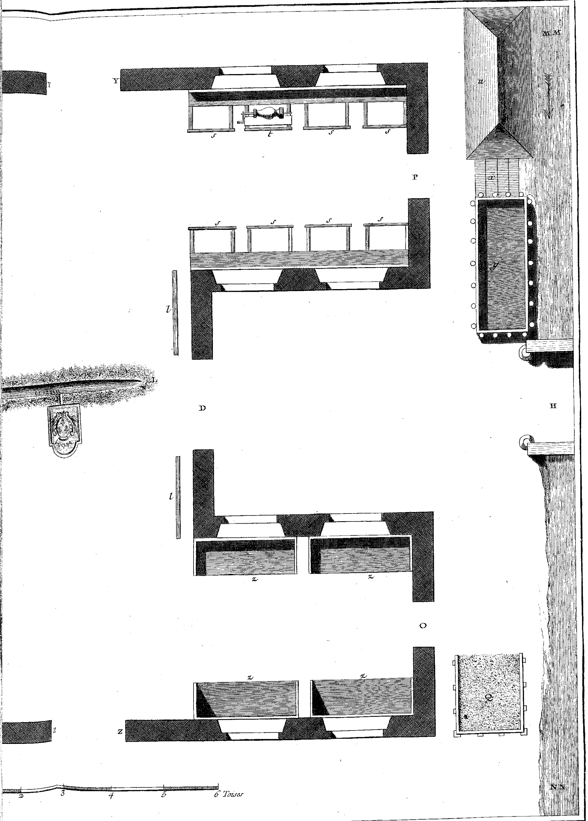
Plan Général d'un Fourneau en Marchandise.
