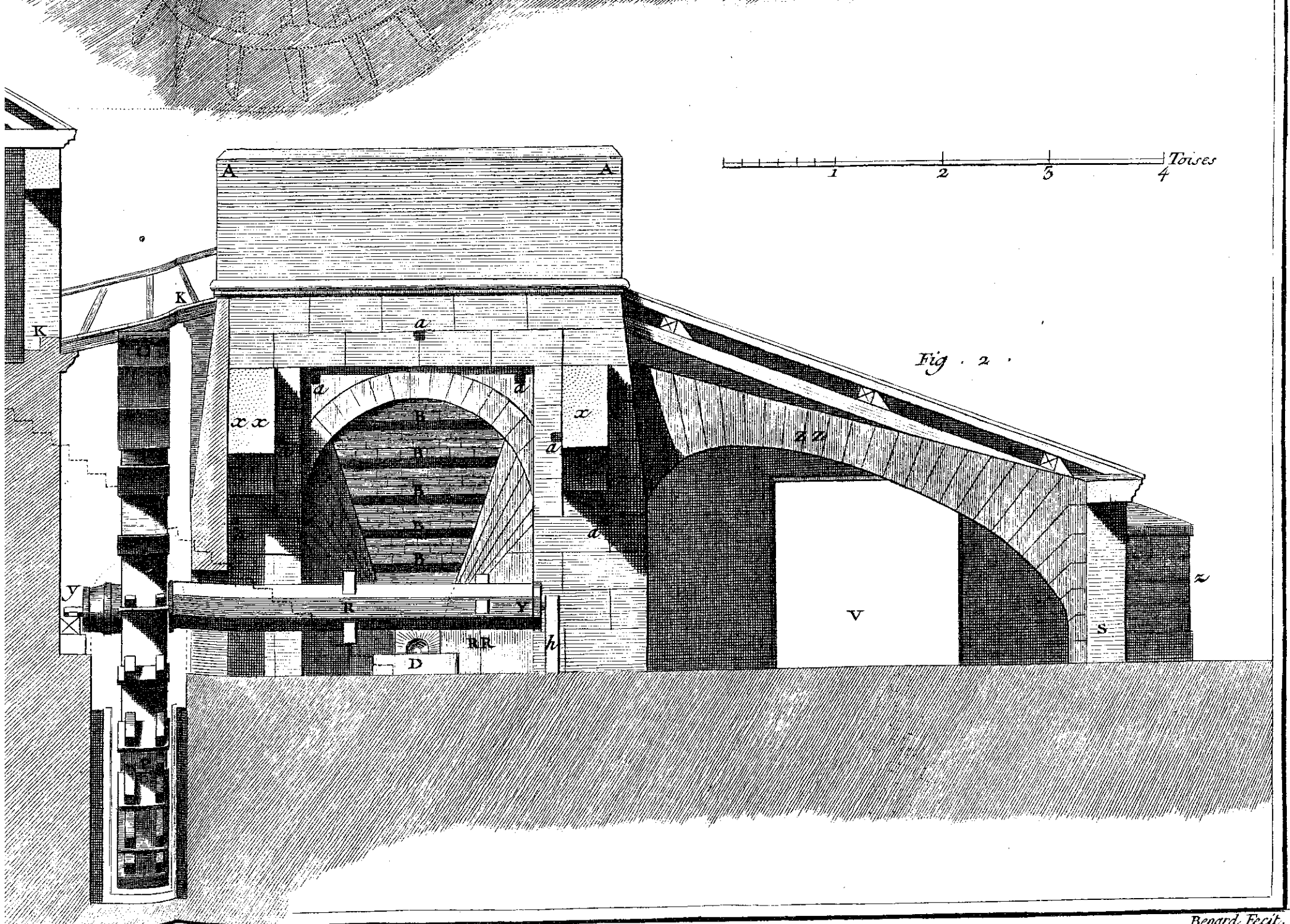
Fourneau à Fer, Elevations et Coupes d'un Fourneau.
