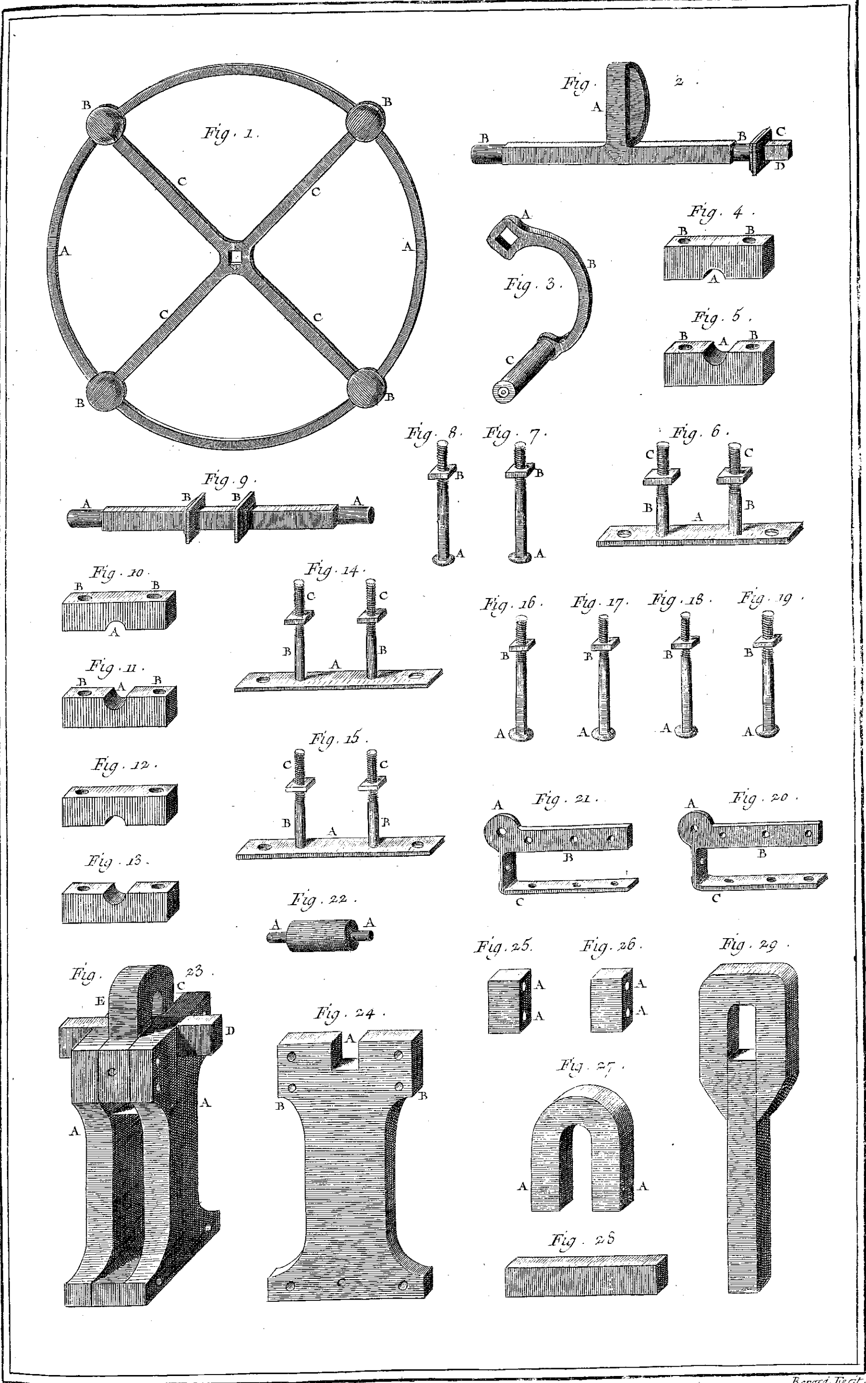
Serrurerie, Détails du martinet à bras et de l'Étau à moufles.
