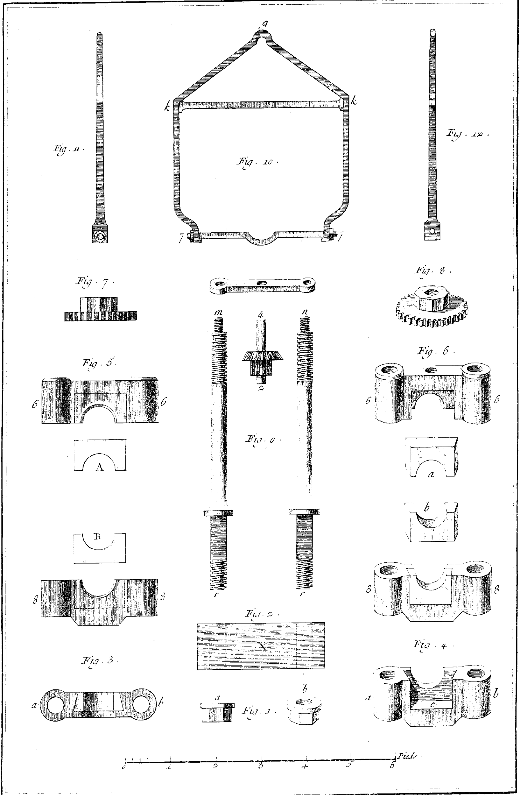
Laminage du Plomb, Développemens des Pièces qui composent la garniture d'un des cotés du Laminaire représenté dans la Planche précédente.
