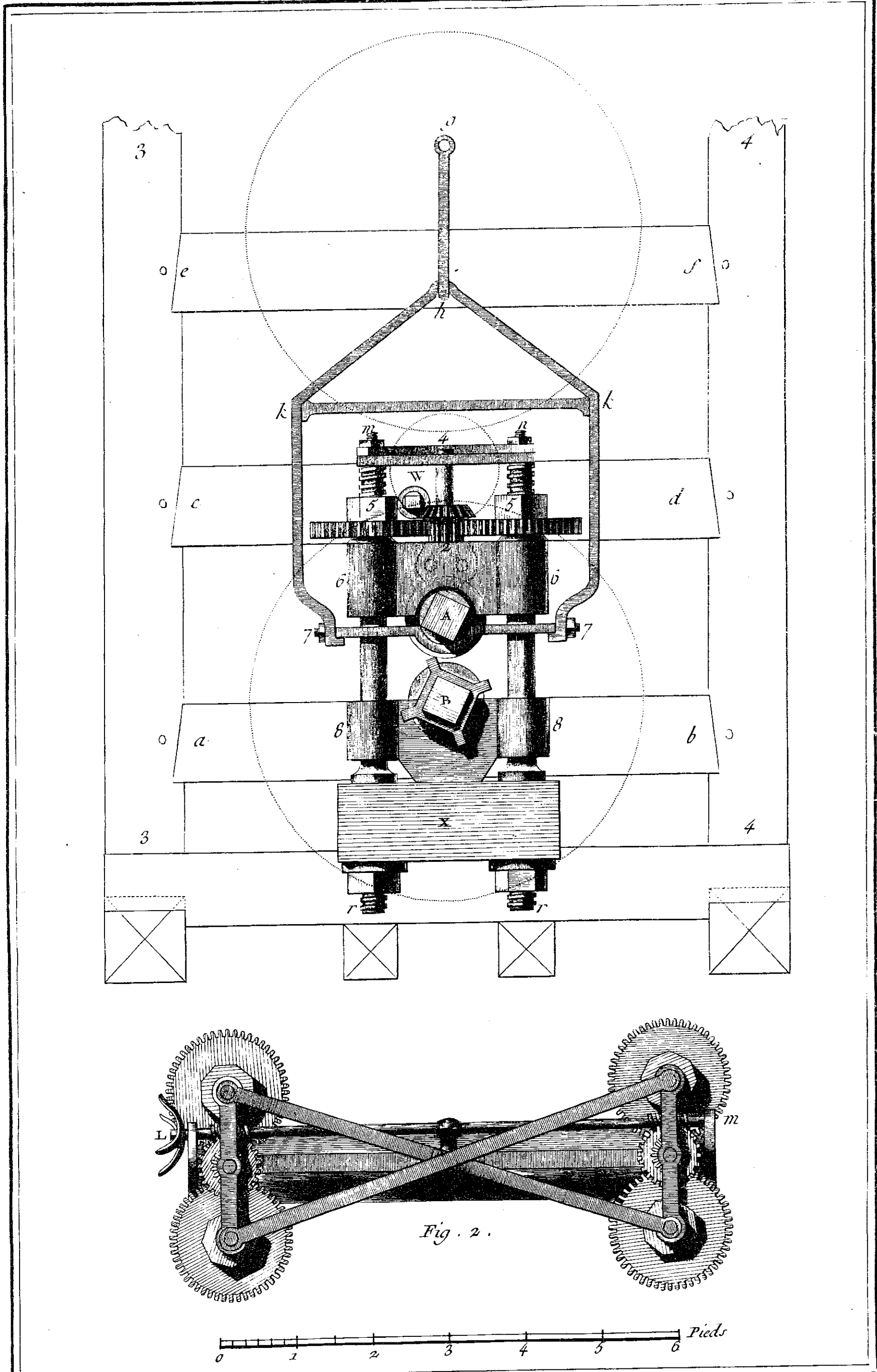
Laminage du Plomb, Élévation Latérale d'un Laminoir et Plan du Régulateur.
