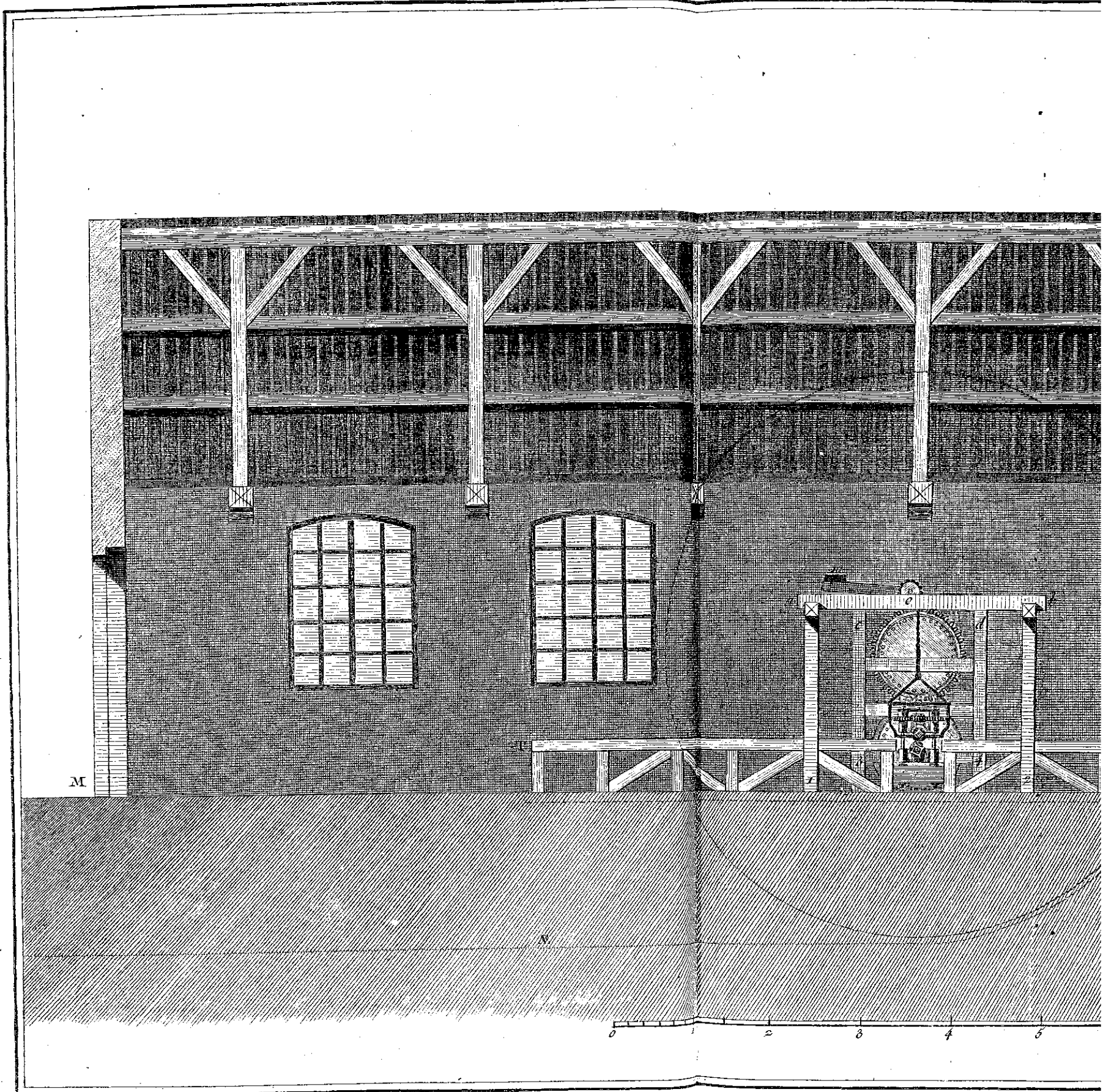
Laminage du Plomb, coupe Longie
