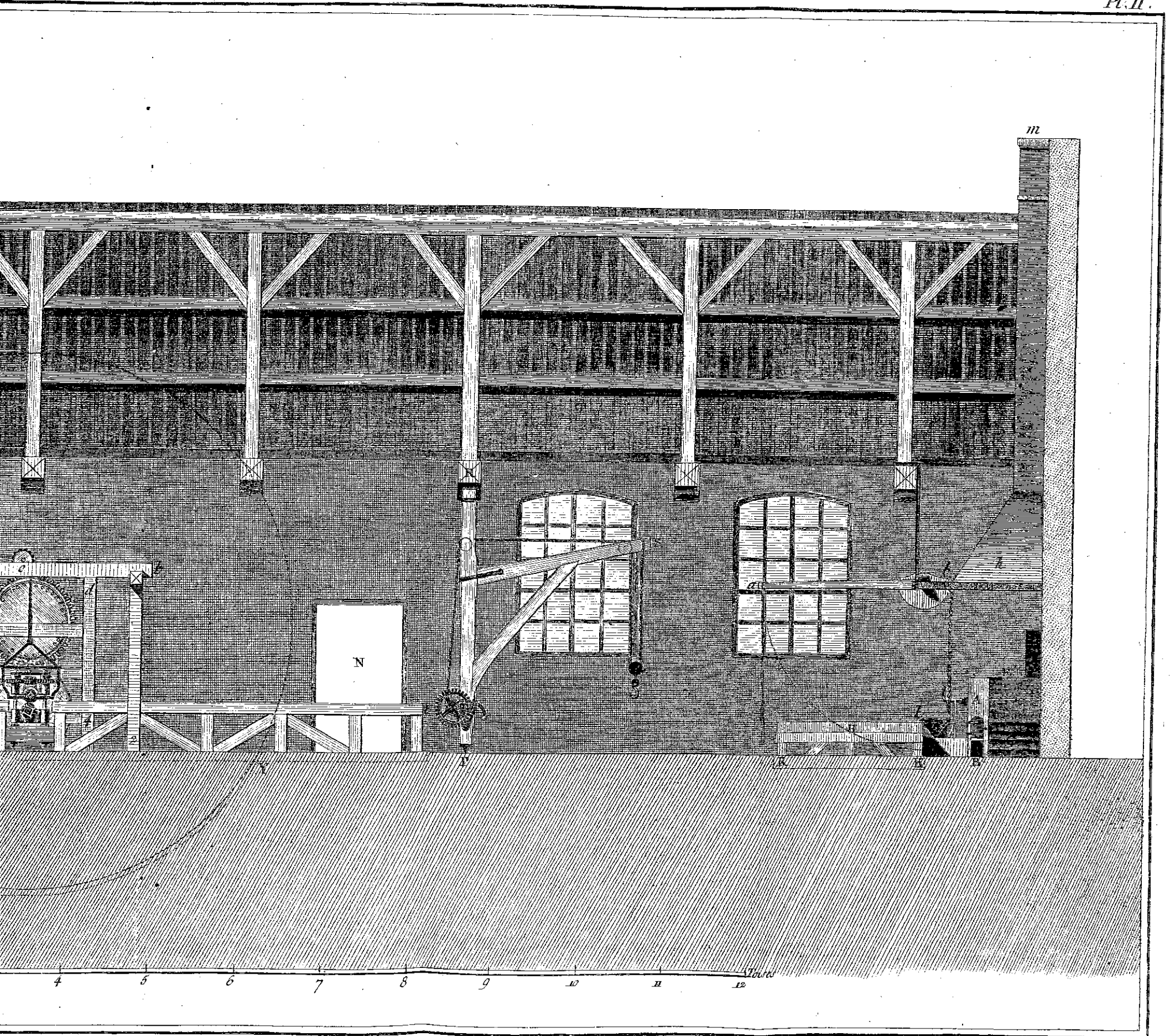
Coupe Longitudinale de l'Atelier du Laminoir.
