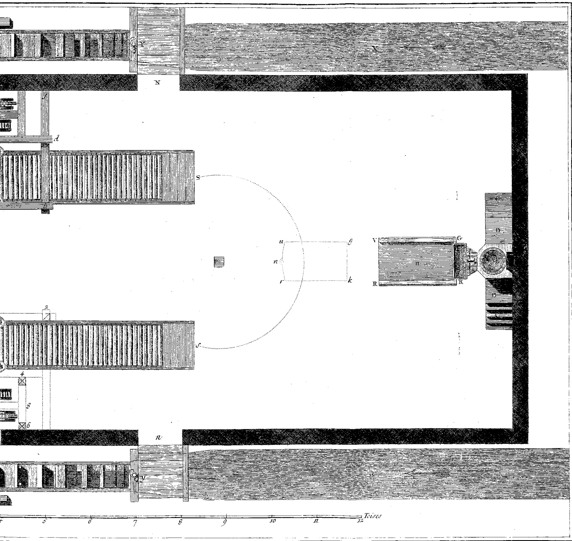
Plan général de la Fonderie et des deux Laminaires.
