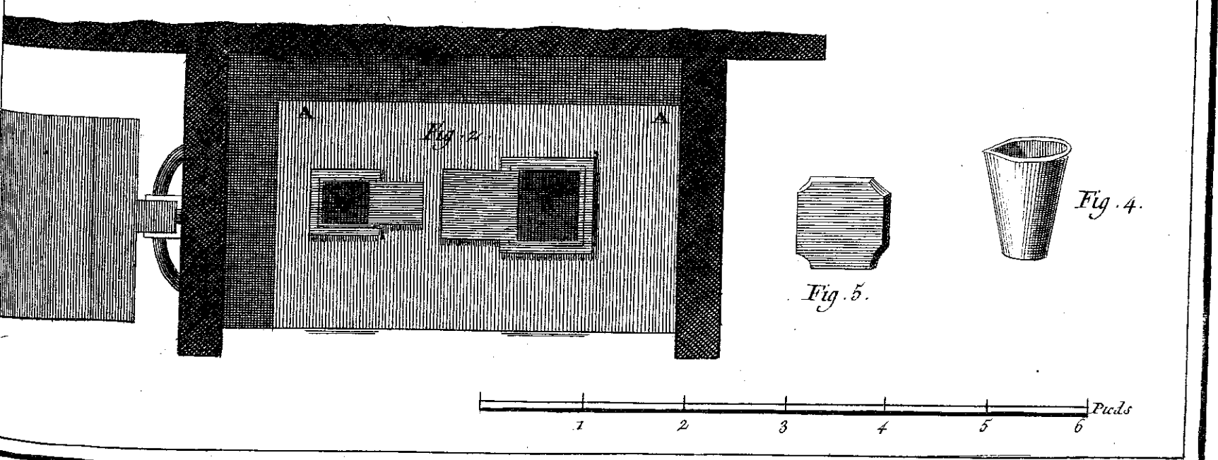
Monnoyage, Fourneau a Soufflet pour l'Or.
