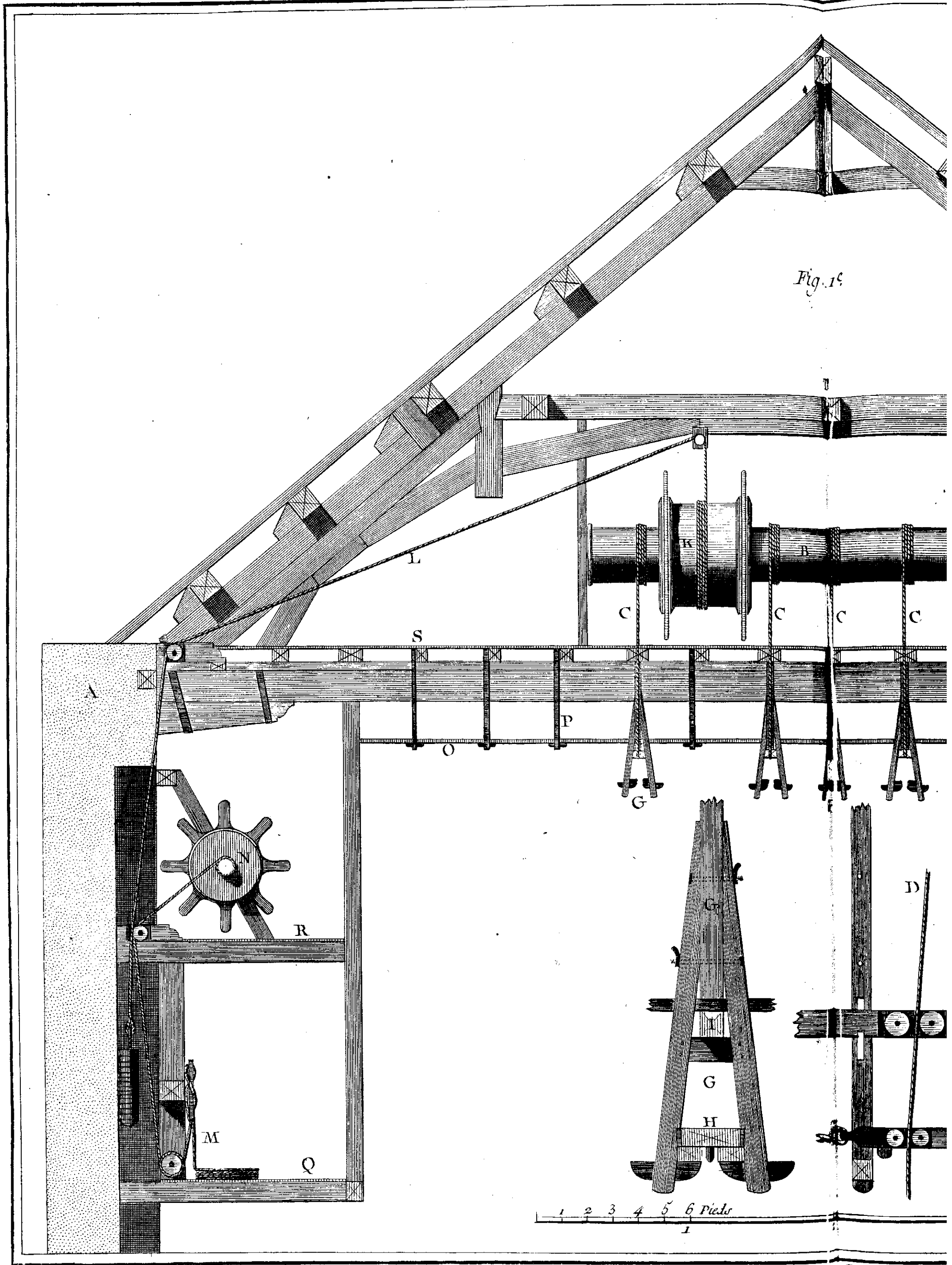
Machines de The Élévation en Coupe de la Charpente en travers des Fermes et Corridors avec le Développement d'une Ma
