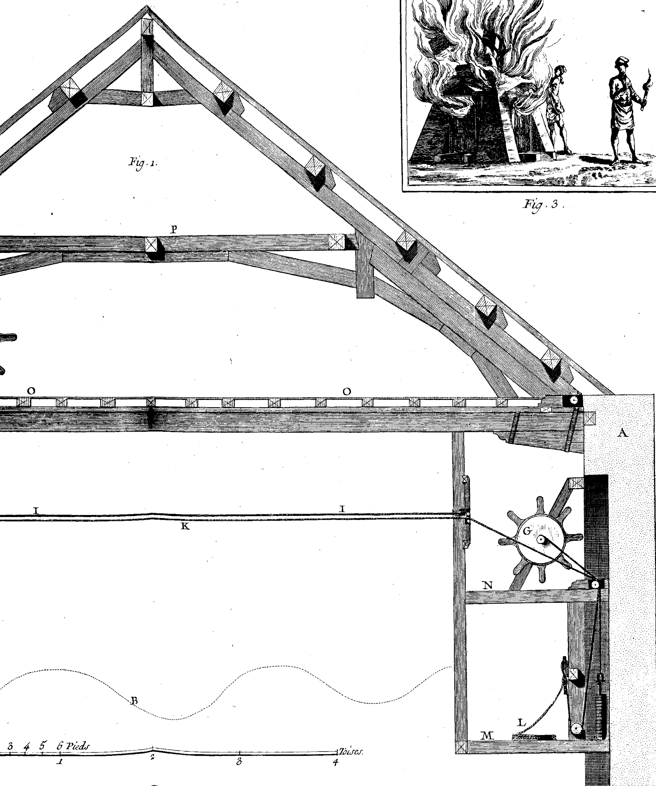
Machines de Theatres, Machine du Chemin ceintre et idées ou esquisses de Décorations d'un Salon dans lequel Médée poignarde ses enfans à Jason, et démolition d'un Tombeau enflammé avec le Service des éclairs.
