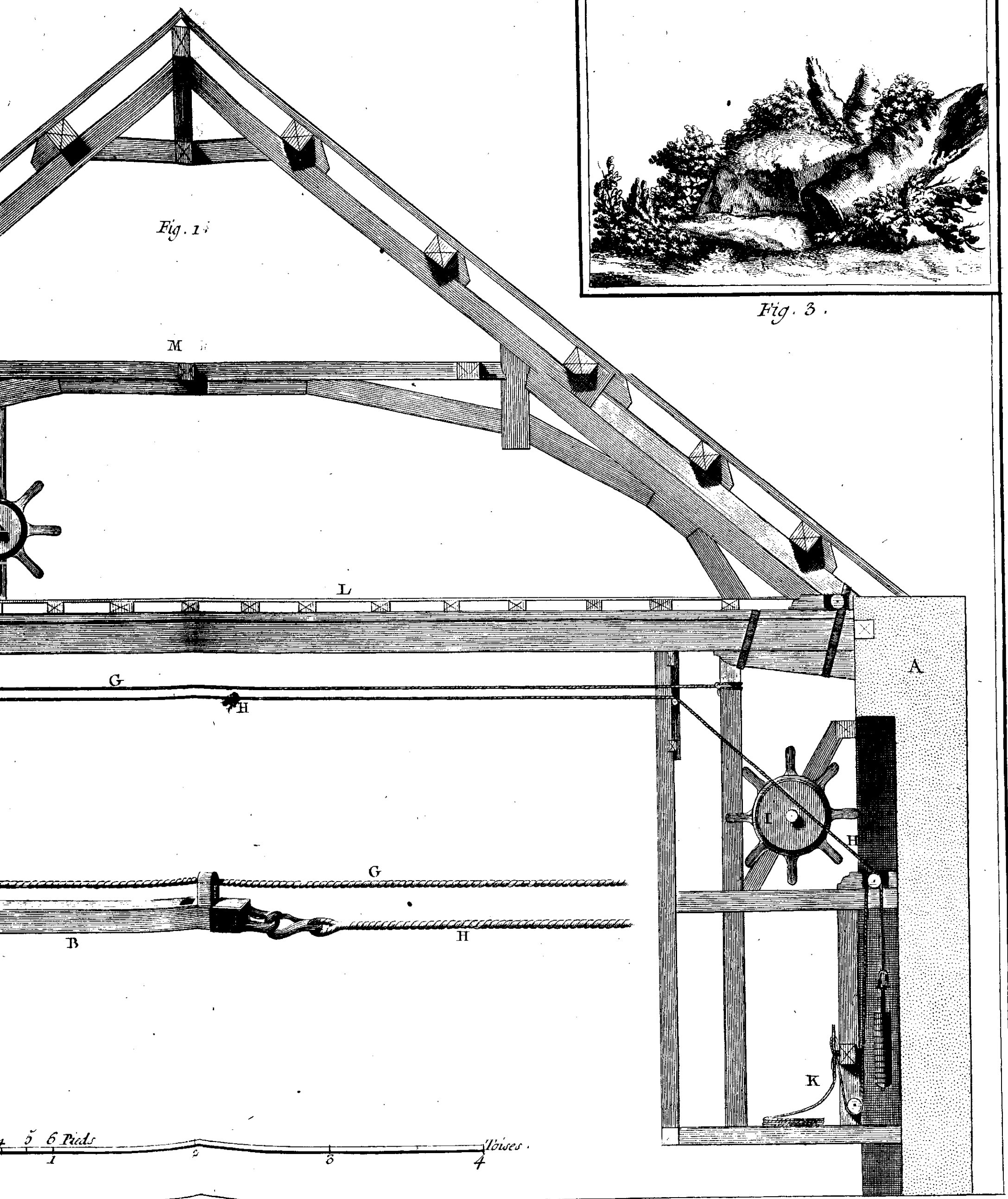
Machines de Théâtres, Machine de travers montant du Théâtre au ceintre; et idées ou esquisses de Décorations d'une Forest et de un Banc de tronc d'arbre et de gazon servant dans la meme Décoration.
