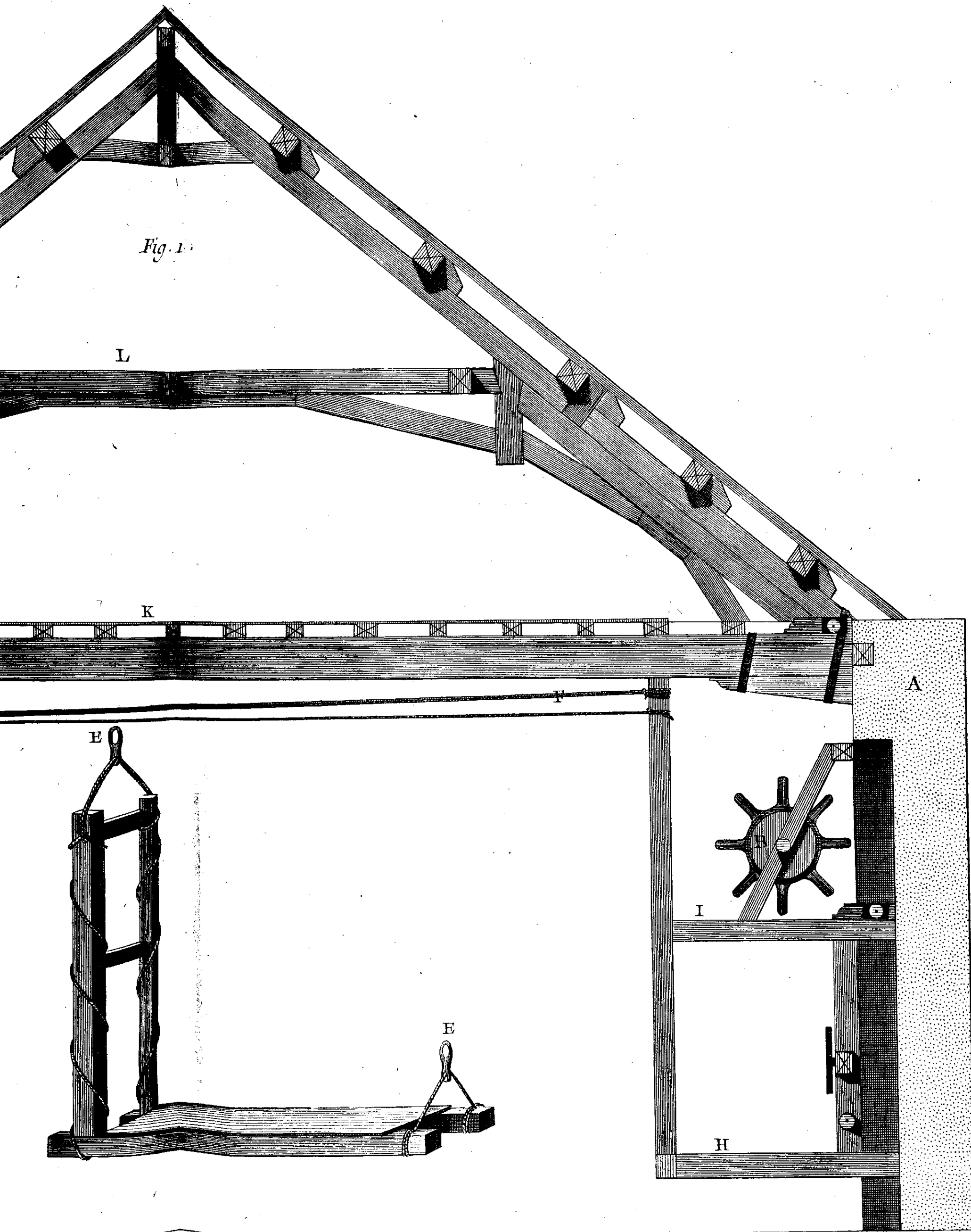
Machines de Théâtres, et le Service et Développement de la Machine pour descendre un Acteur d'un côté du Théâtre à l'autre côté.
