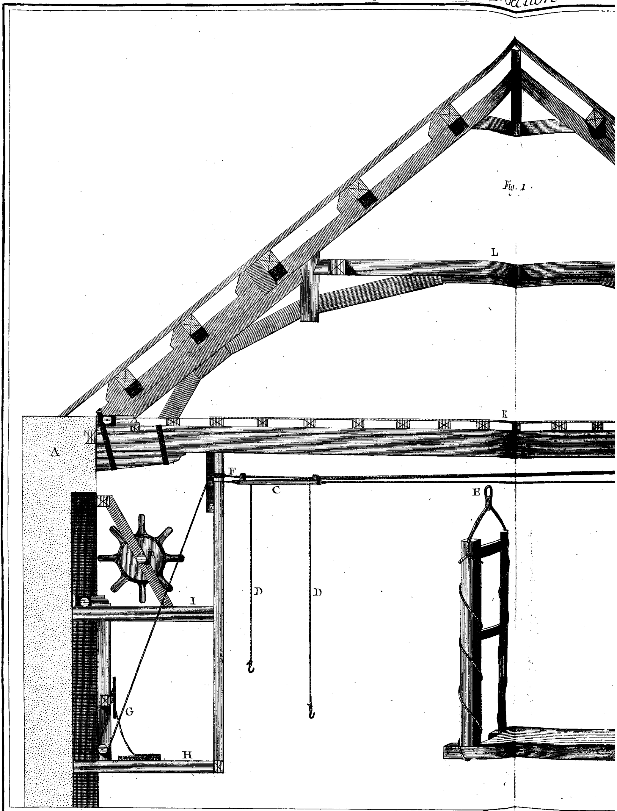
Machines de Théâtre Élévation en Coupe de la Charpente du Comble et des Corridors, avec le Service et Développement de la M
