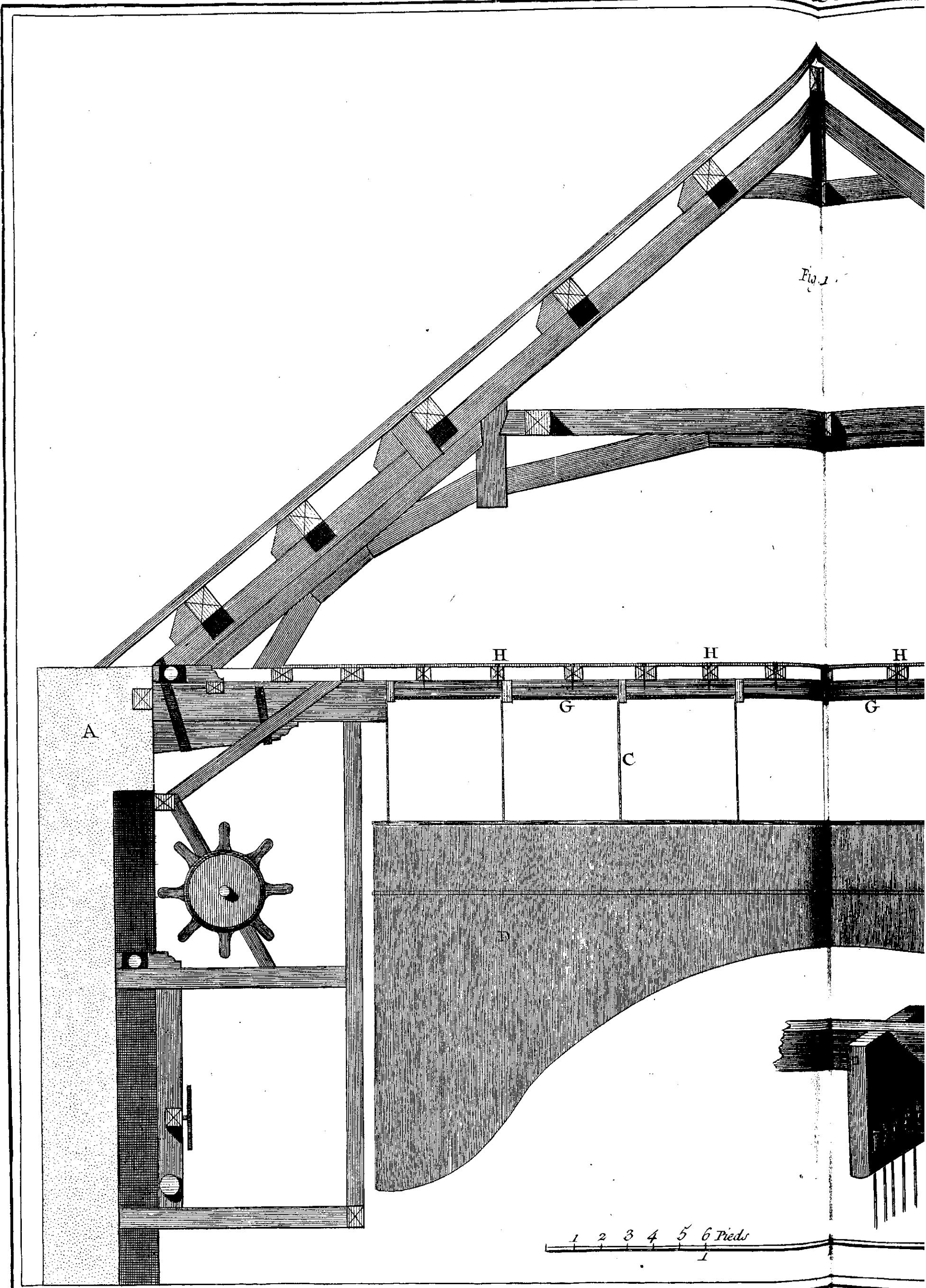
Machines de The Elévation sur la largeur du Théâtre avec les Treuils pour le Service des changemens et des ci
