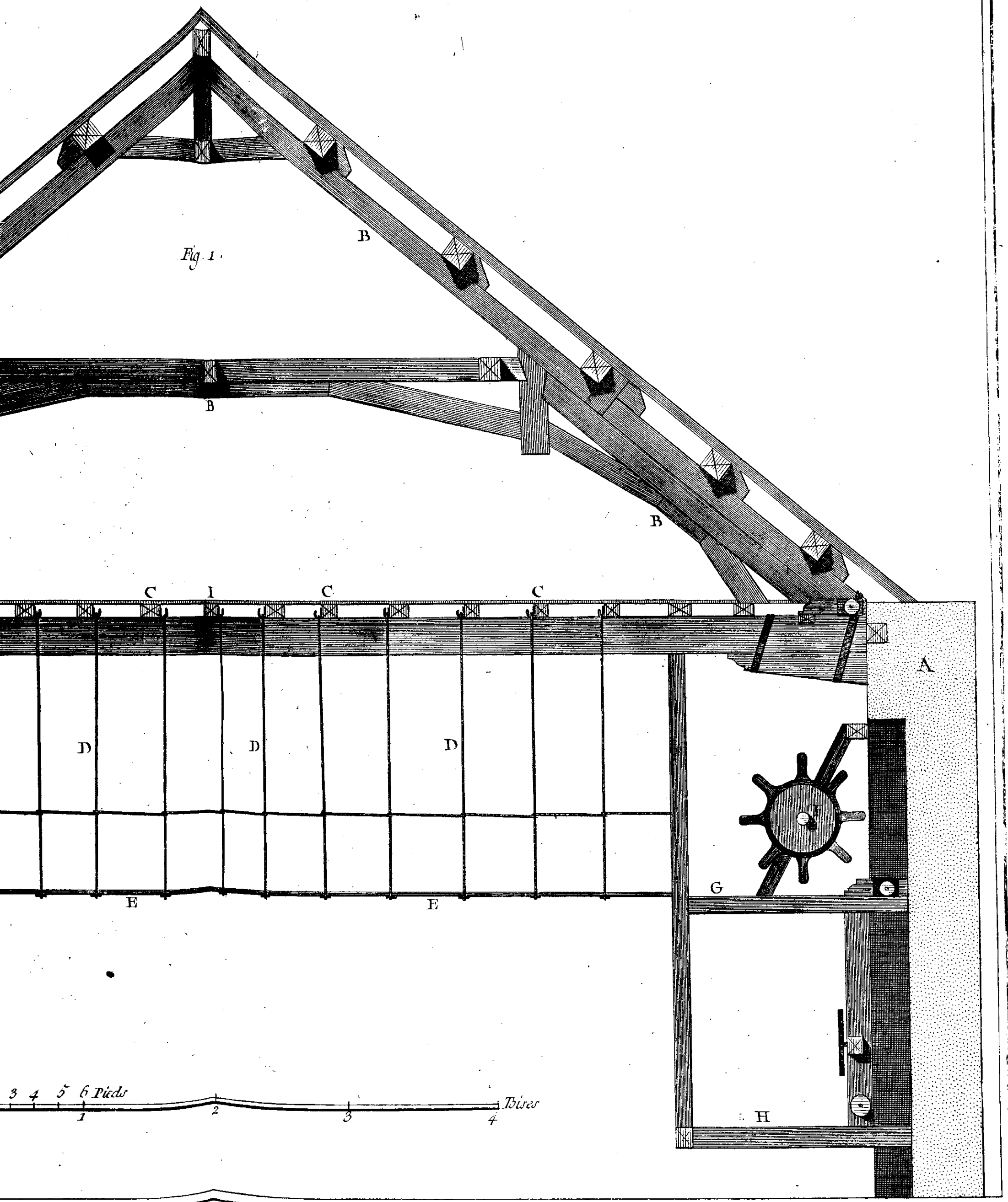
Machines de Théâtres, Tréuils, les Contrepoids, et les Ponts de communication d'un Corridor à l'autre soutenus par des Étriers de cordages accrochés sur des solives.
