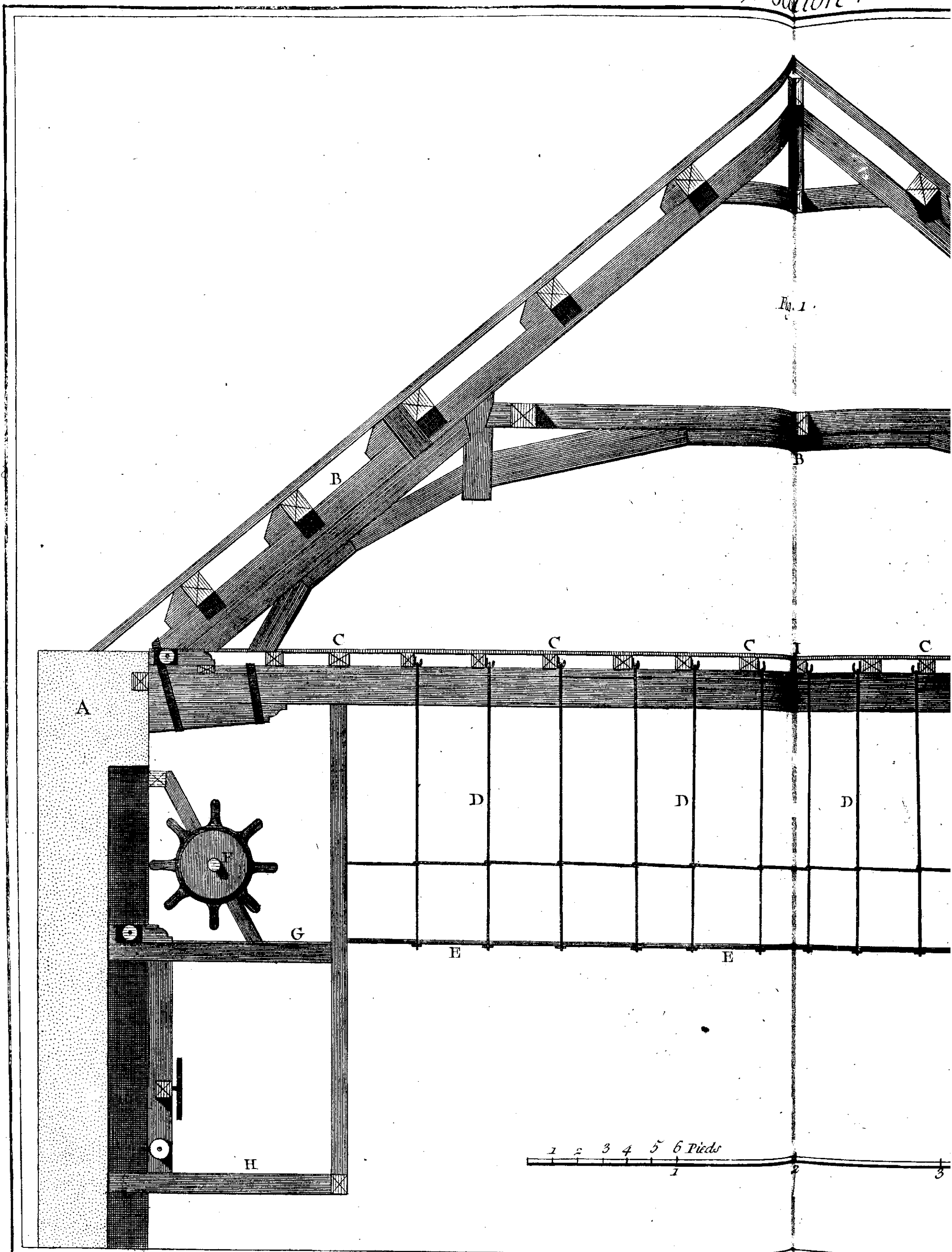
Machines de Théâtre Élévation en Coupe sur la largeur du Théâtre, avec les Corridors, les Treuils, les Contrepoids et les Ponts de communication
