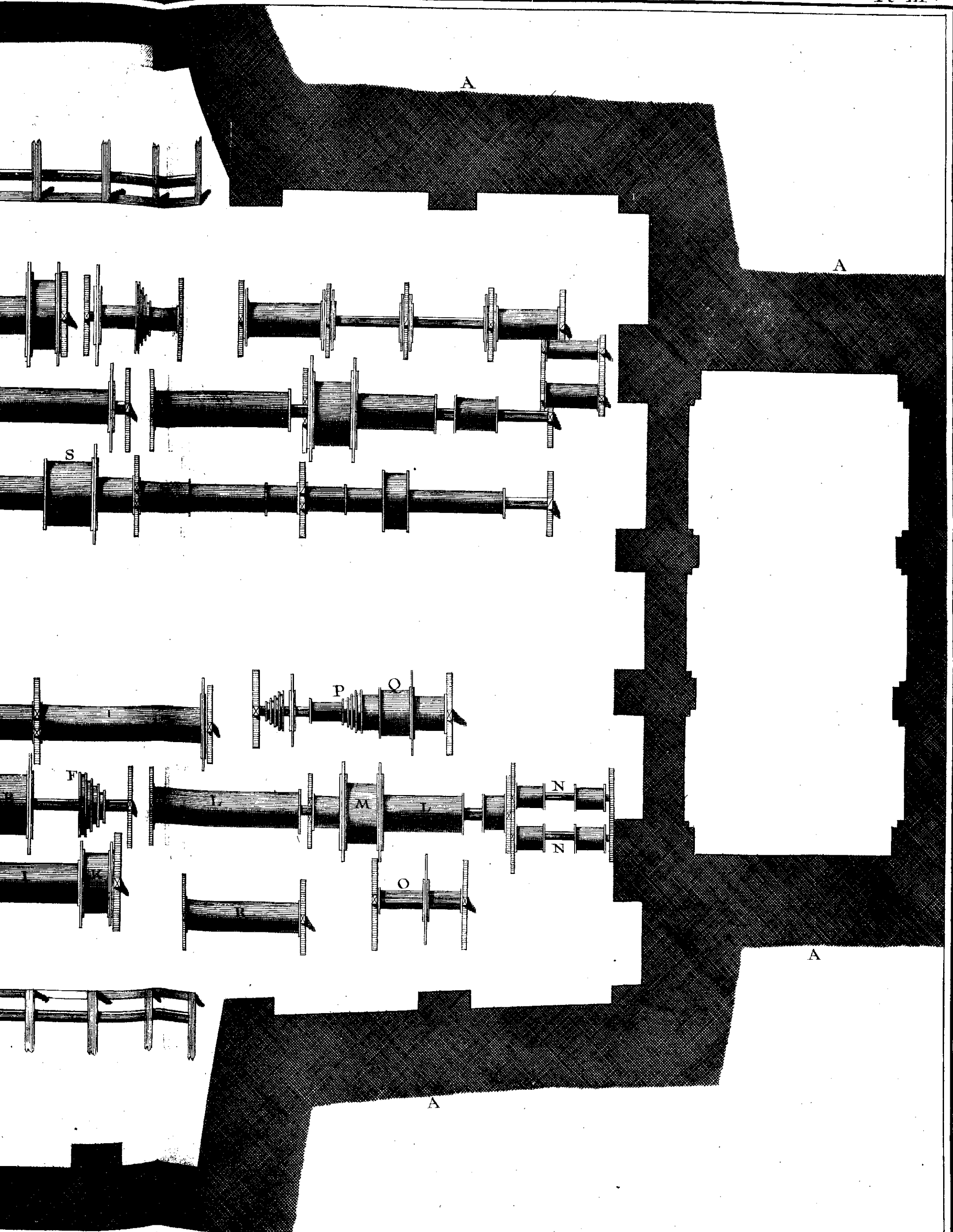
Machines de Théâtres. et de gradés et des Treuils employés au Service des Machines du Ceintre.
