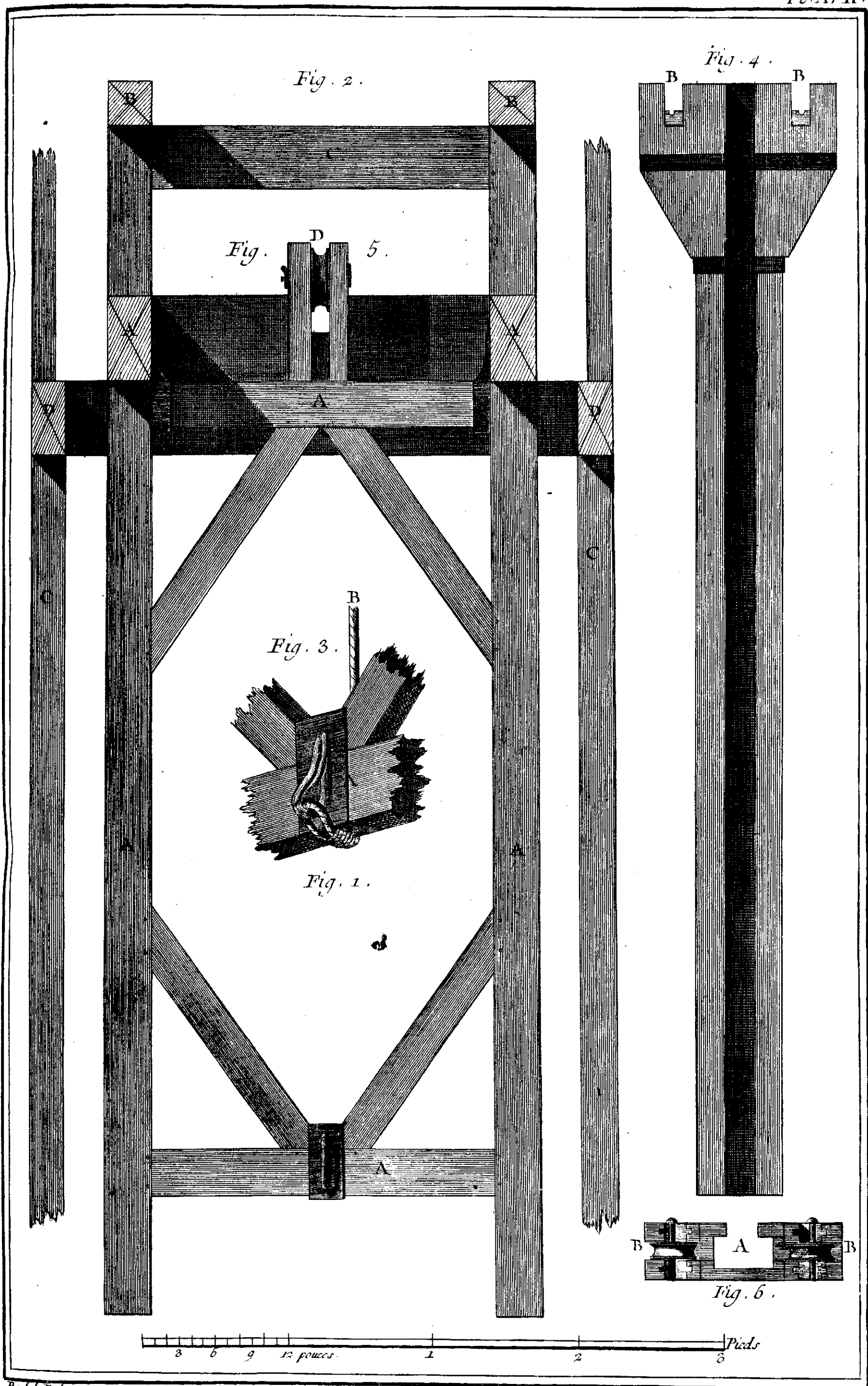
Machines de Théâtres, Élévation Géométrale des Batis servant d'aune pour monter les Chemins centrés avec leurs Equipages.
