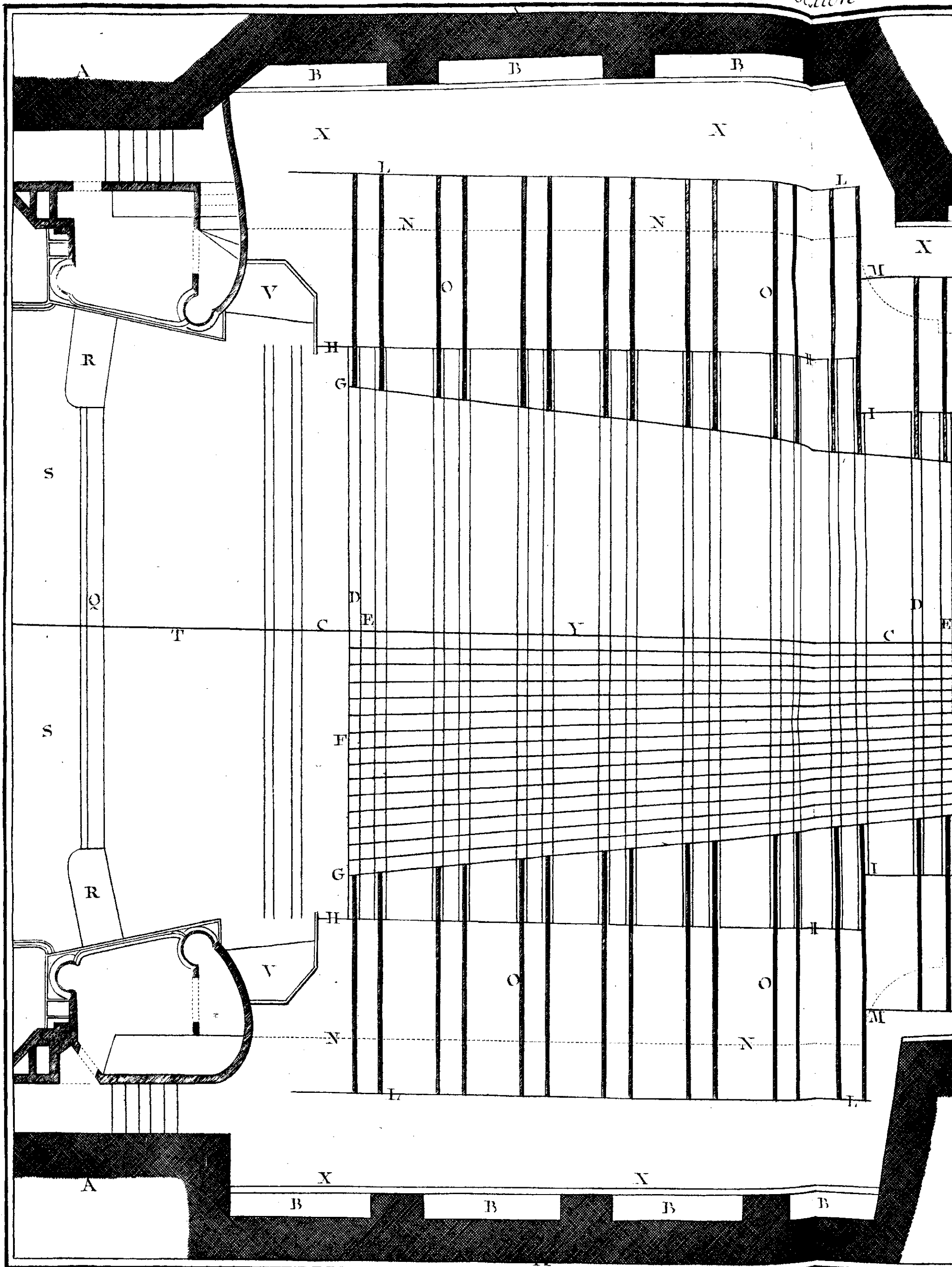
Machines de Théâtre Plan du Théâtre au niveau des Décorations, et Distributions des Trappes
