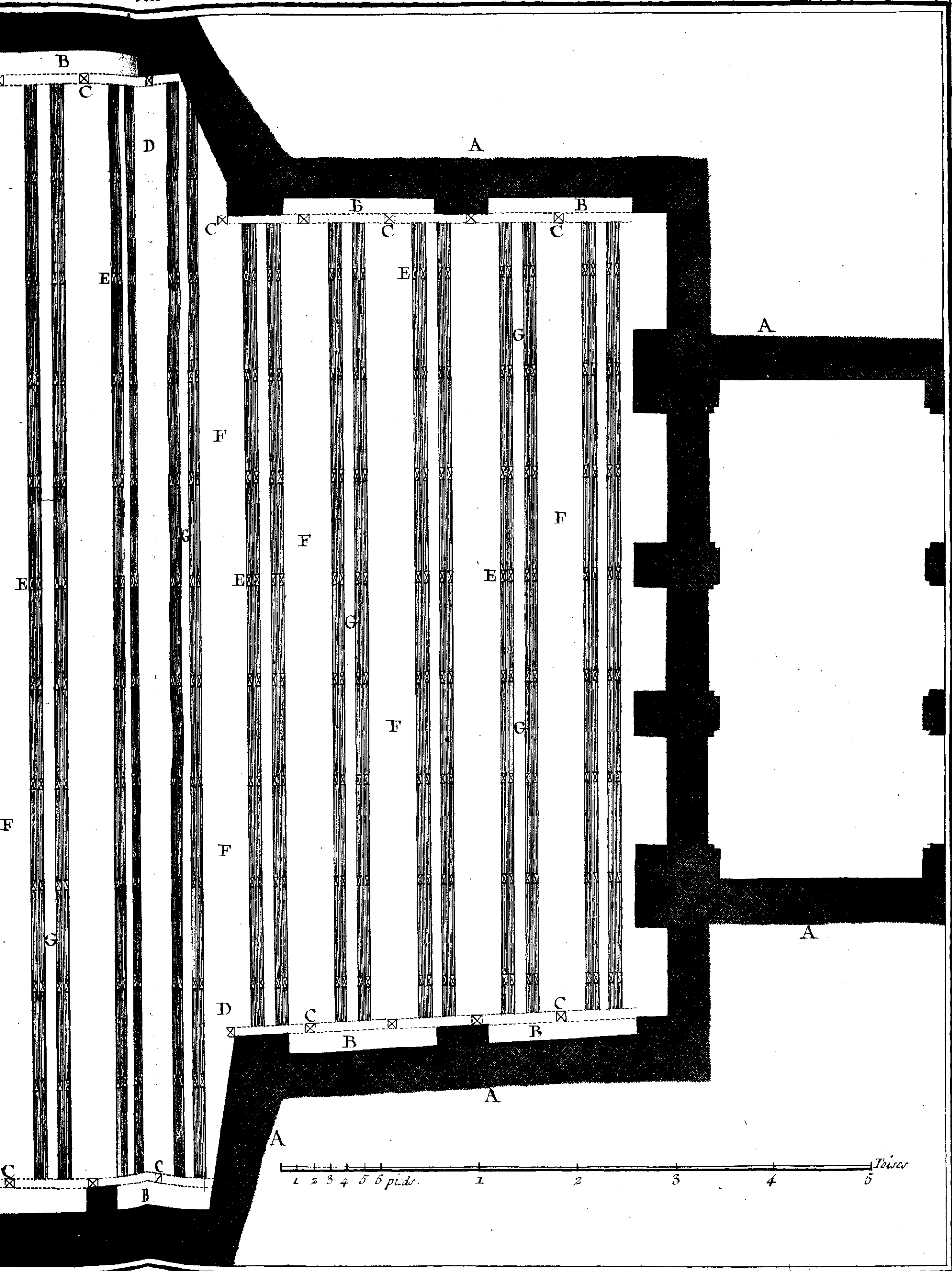
es, Plan du premier dessous pris au dessus des Tambours.
