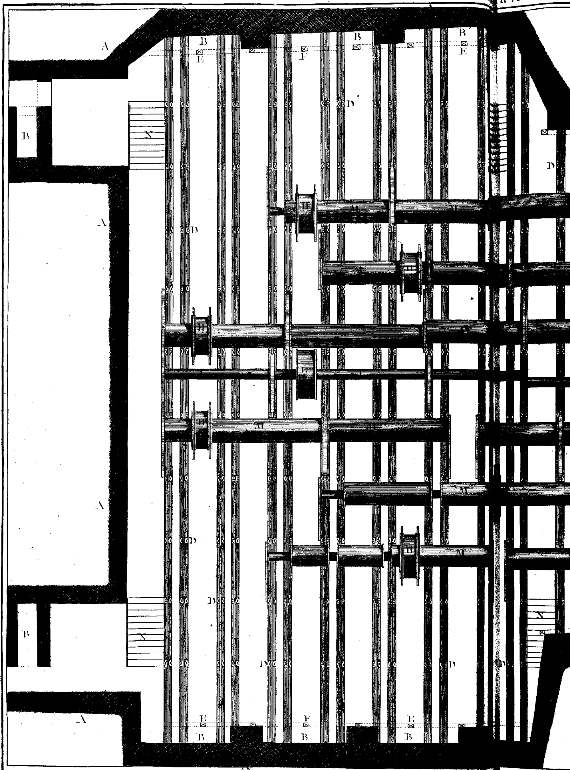
Machines de Théâtre Plan Général des Plattes formes posées sur les Parpins susdits, et Plan des Tambours
