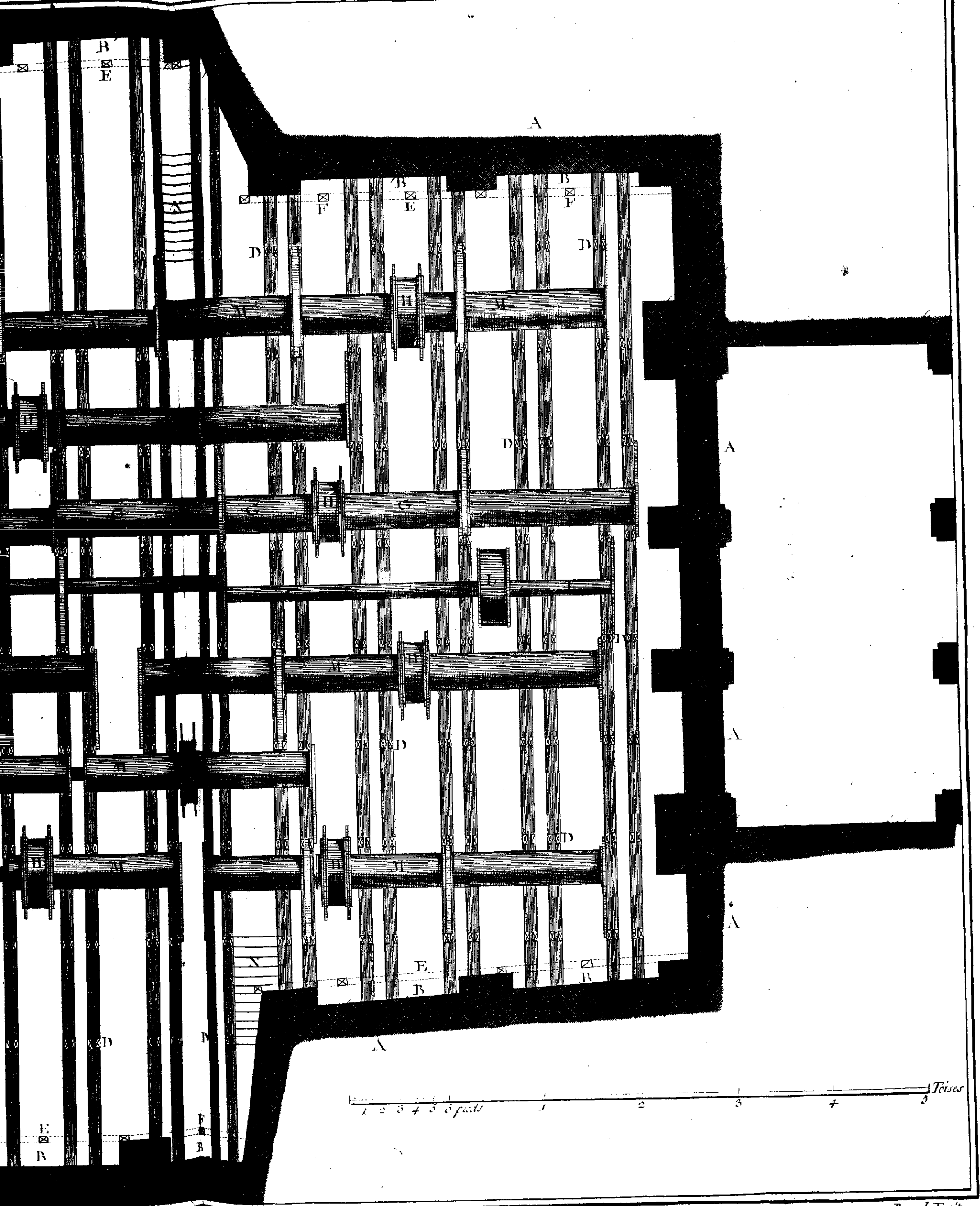
Machines de Théâtres. susdits, et Plan des Tambours servants généralement pour tous les changements de décorations.
