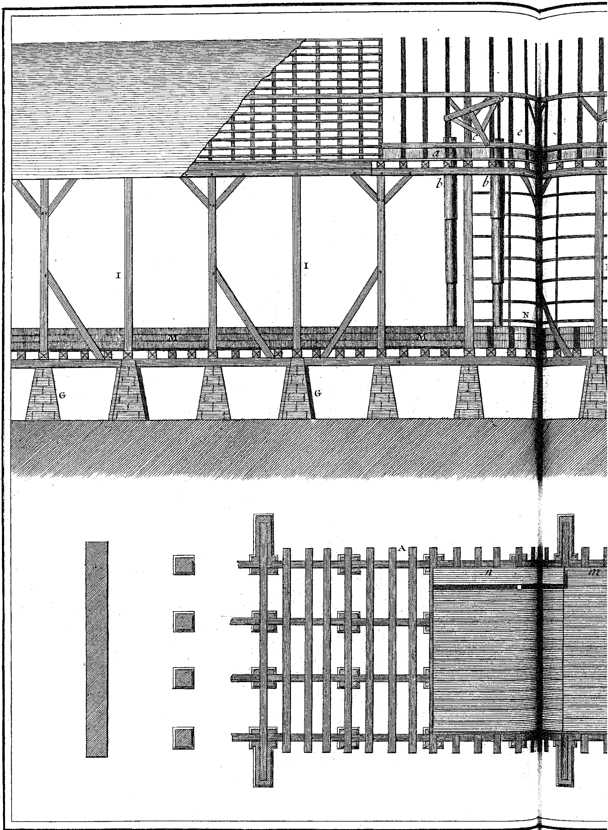
Minéralogie, salines, Plan et Élévation d'une partie des Bâtimens et Platte forme Supérieure où sont les Chesneaux qui
