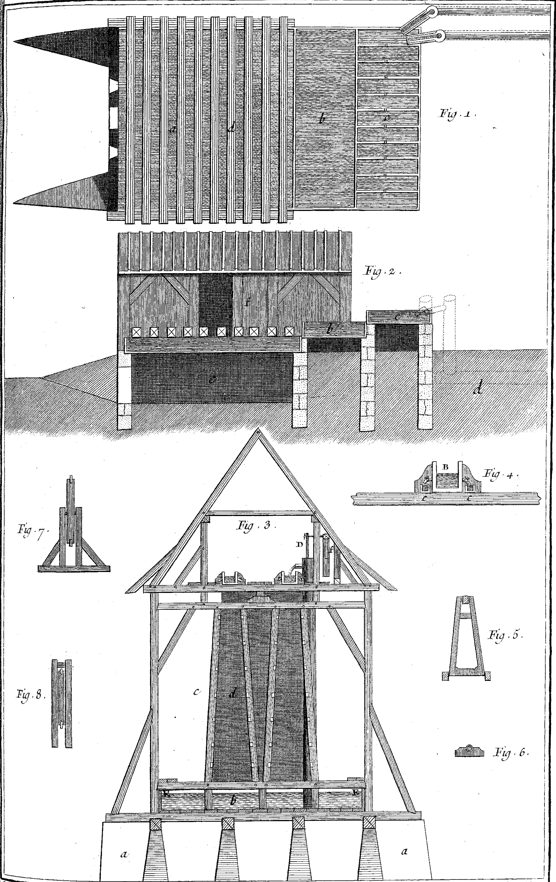
Minéralogie, salines. Plan et Profil d'une Poêle de Roxieres et Développemens.
