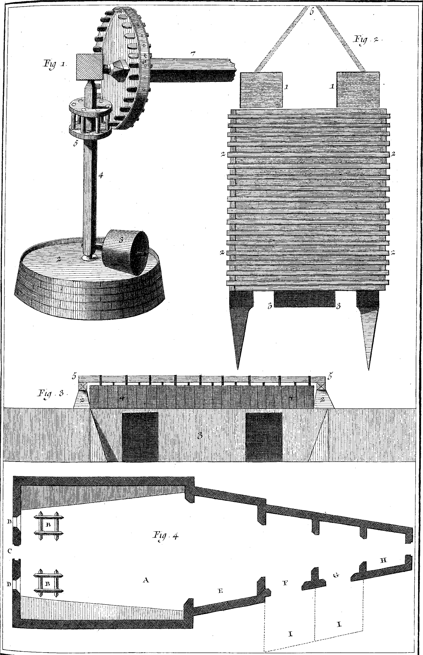
Minéralogie, Salines, Plan, Profil et Élévation des Poësles de la Saline de Dieuze et Plan d'une nouvelle Poësle avec ses Poësillons établie en 1738 à Dieuze et Chateau Salins.
