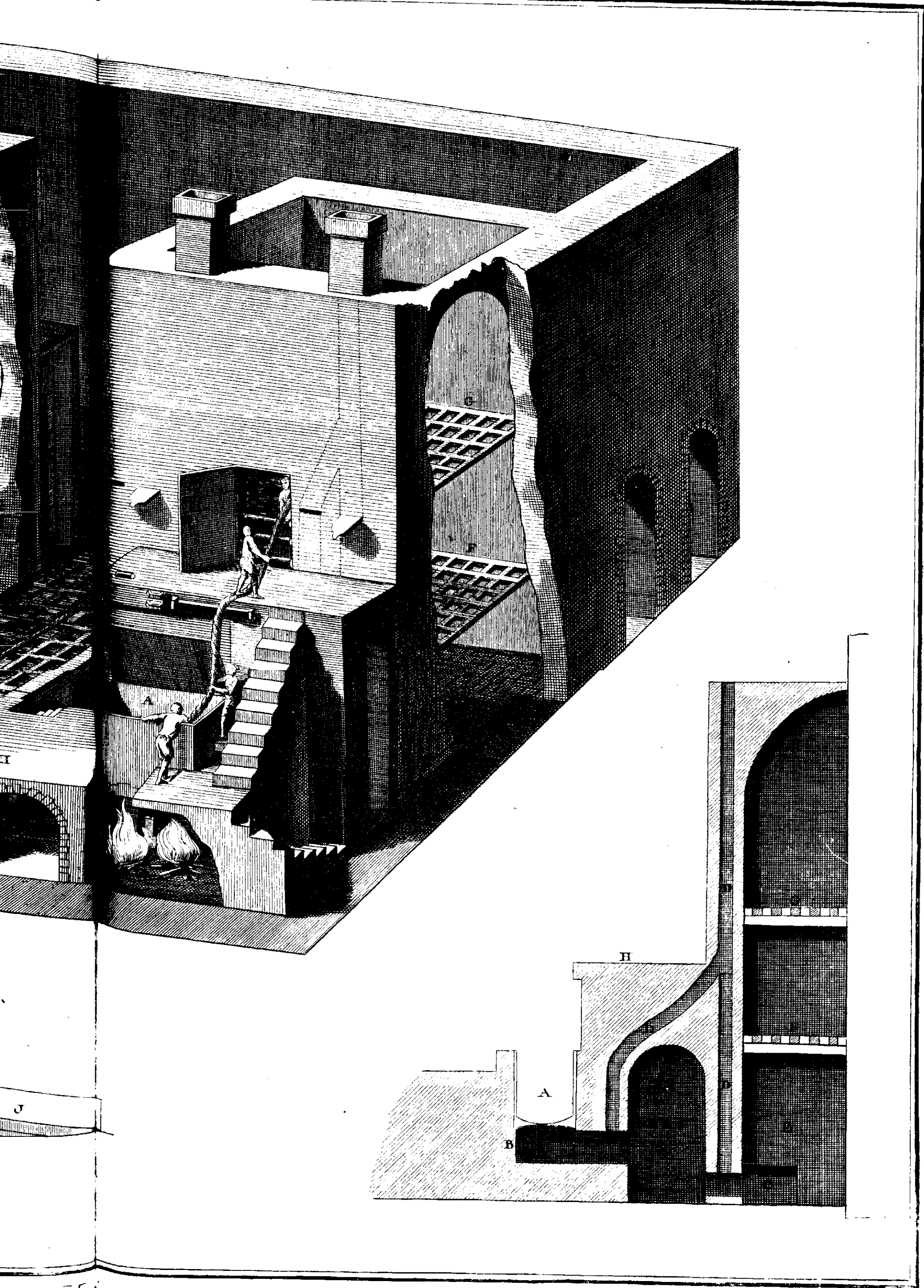
Matte, u Plan de la Planche X. avec la vue des Travaux qui s'y font.
