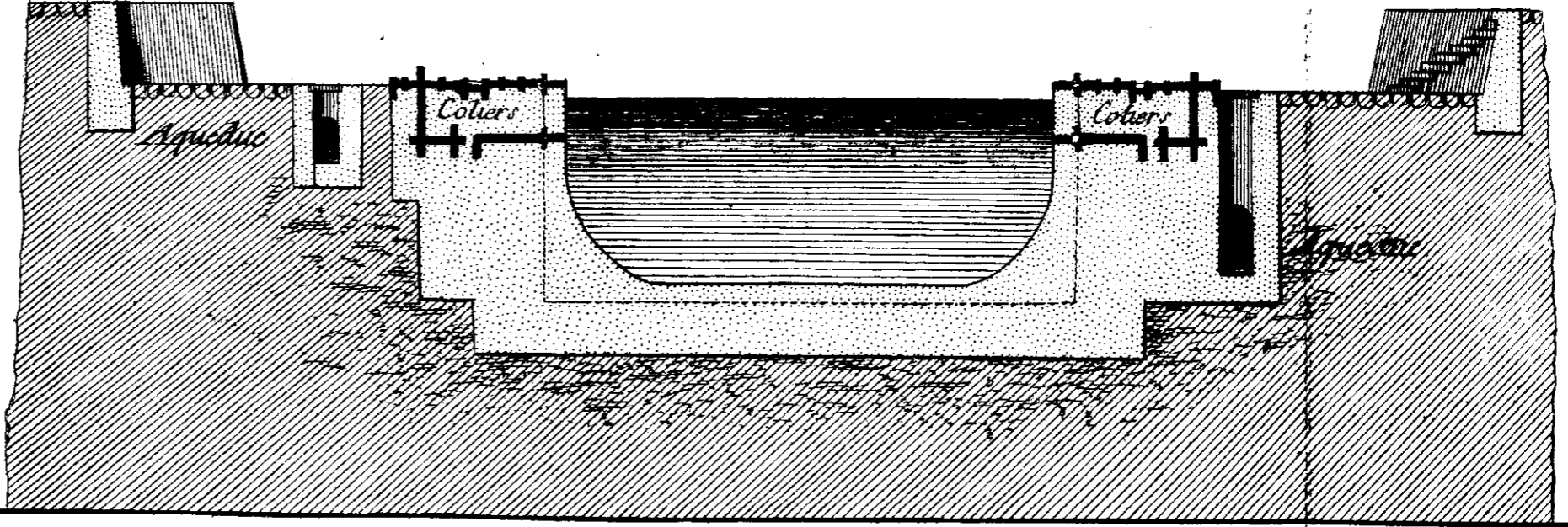
Elevation et Profil des Formes dans leur Longueur Pris sur la Ligne AB.
