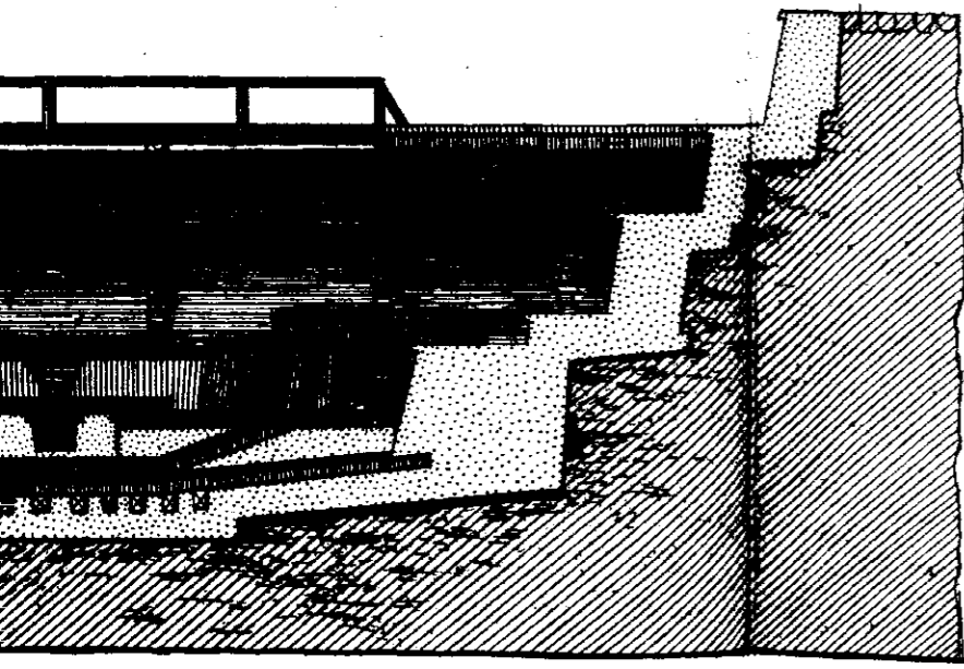
Elevation et Profil des Formes dans leur Longueur Pris sur la Ligne AB.
