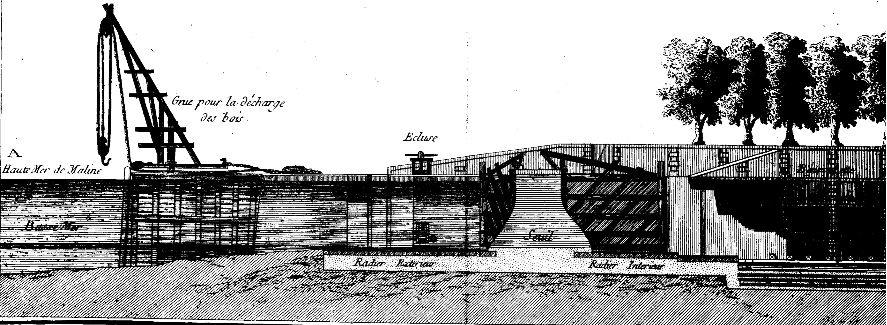
MARINE, Elevations et Profils des Formes de Rochefort et de leurs Diff
