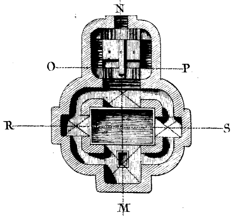
Plan des Galeries du Puits.
