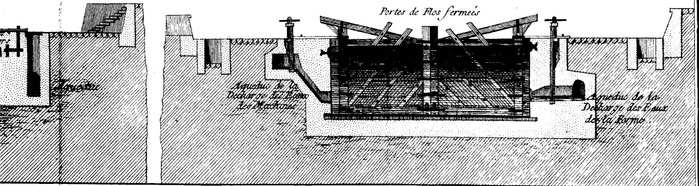
Profil Pris sur la Ligne du Plan I-L.
