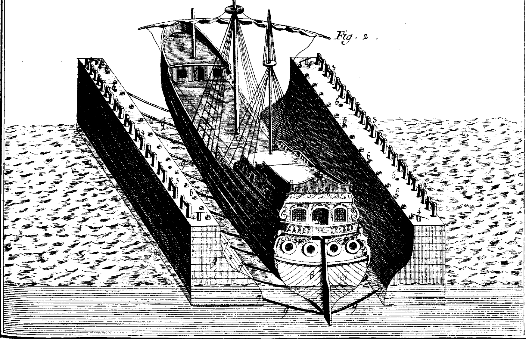
Dessein de la Machine nommée Chameau dont on se sert à Amsterdam pour enlever un Vaisseau.
